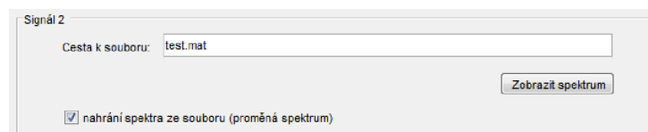
Obr. 4.4: Přímé načtení spektra ze souboru.
