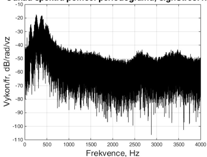
Odhad spektra pomocí periodogramu, signStres7.wav
