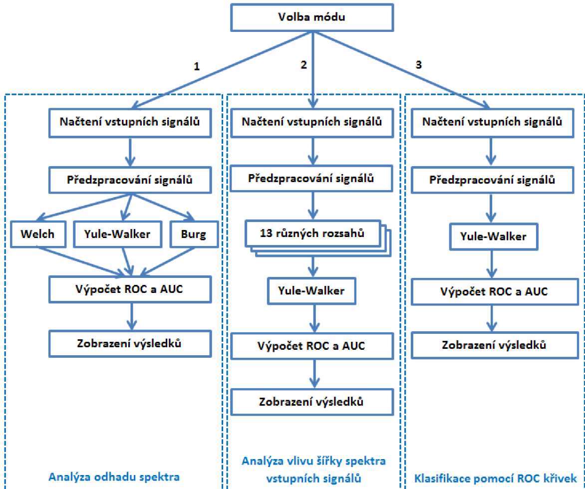
Obr. 4.1: Zjednodušený vývojový diagram programu s předpřipravenými analýzy.
