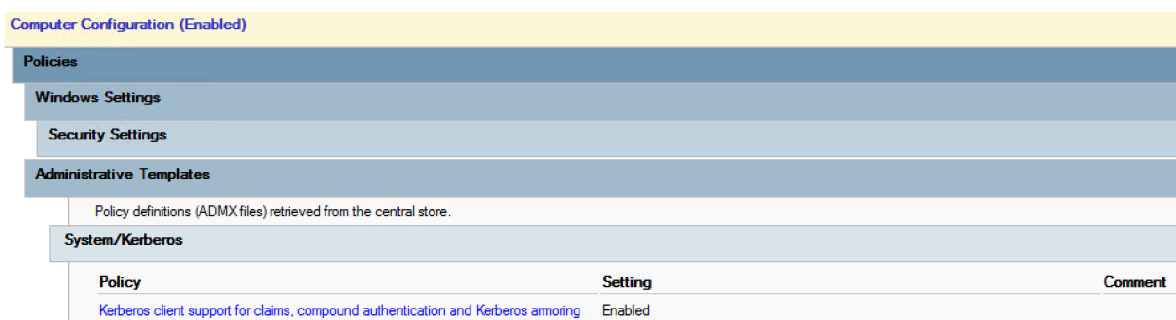
Obrázek 42: Nasazení Kerberos Armoring Default Domain Policy (vlastní)
