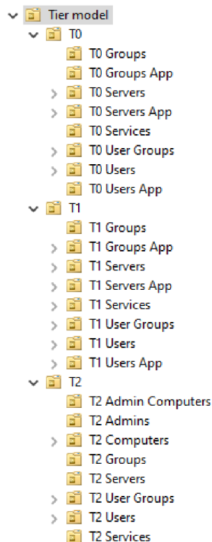
Obrázek 15: Struktura OU Tier Modelu (vlastní)
