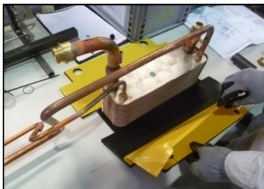
Obrázok 24: Izolácia PHE (Zdroj: Vlastné spracovanie)
