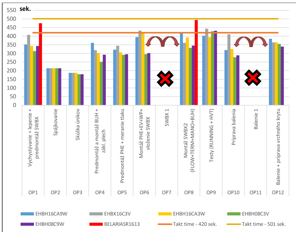
Graf 4: Simulácia výroby - 52 a 62 ks
