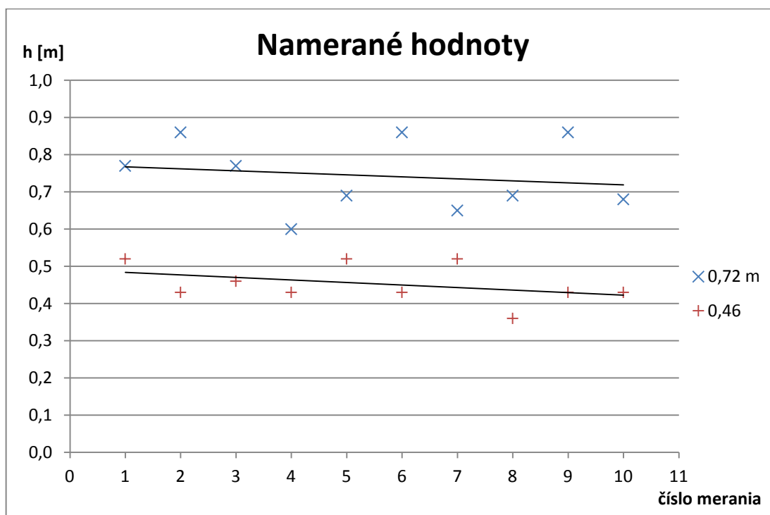
Graf 2 Namerané hodnoty pre čas ustálenia 5 s
