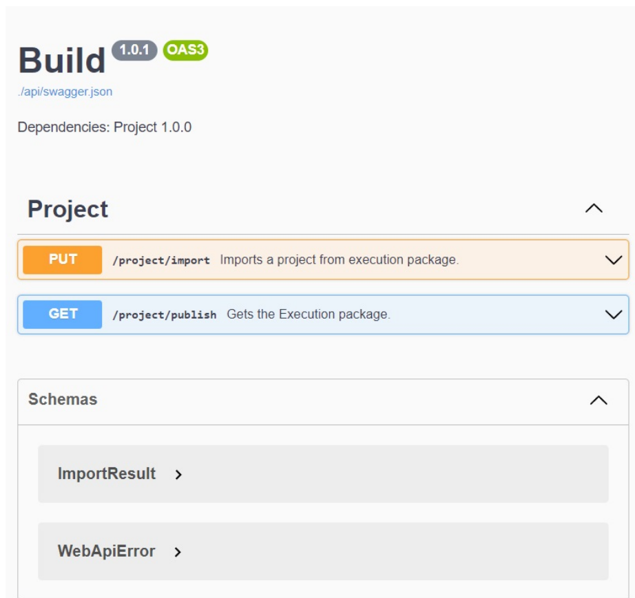
Obr. 3.7: Služba Build
