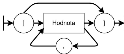
Obr. 2.2: Schéma zoznamu
