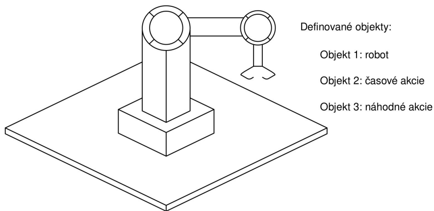
Obr. 3.3: Scéna
