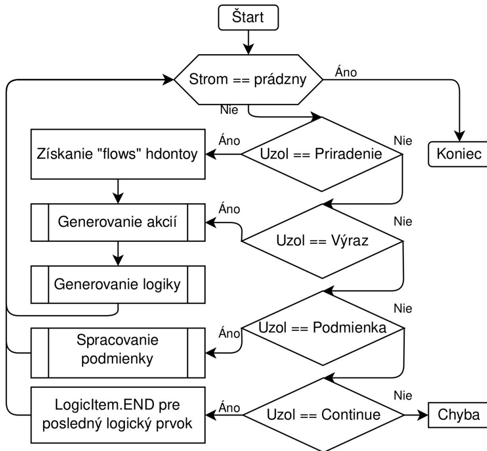
Obr. 4.1: Prechádzanie stromu
