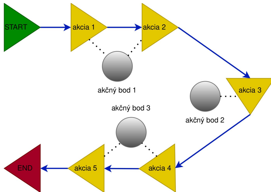
Obr. 3.4: Projekt
