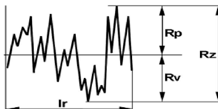
Obr. 3.9 Profil obrobenej plochy se znázorněním Rz [31].
