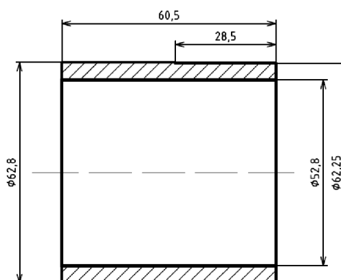
Obr. 3.1 Náčrt obrobeneho vzorku.
