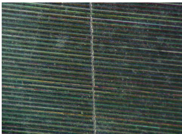
Obr. 3.28 Detail praskliny vzniklé při obrábění vzorku číslo 32.
