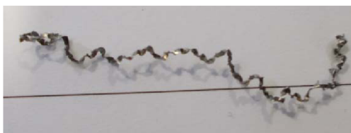
Obr. 3.27 Tříška odebraná během obrábění vzorku 37.
