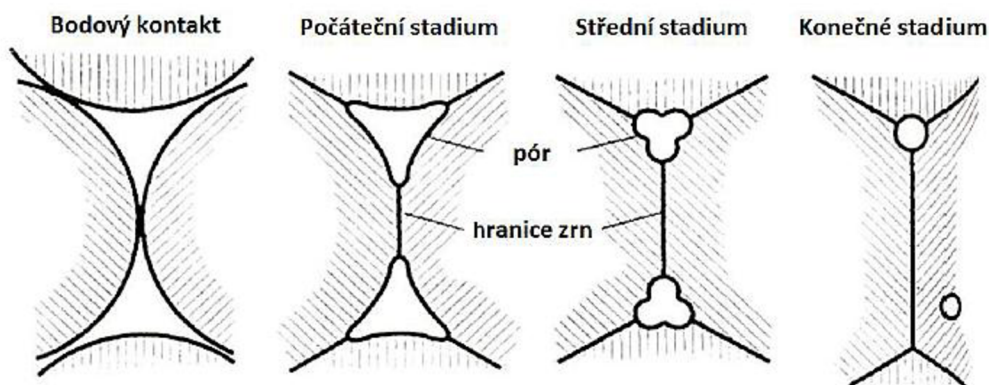
Obr. 2.10: Snižování objemu pórů v průběhu slinování [5]
