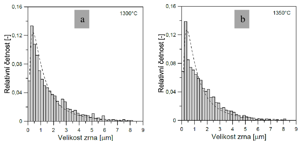
Obr. 5.16: Distribuce velikosti zrn TiB 2 ve vzorku slinutém a) při 1300 °C, b) při 1350 °C
