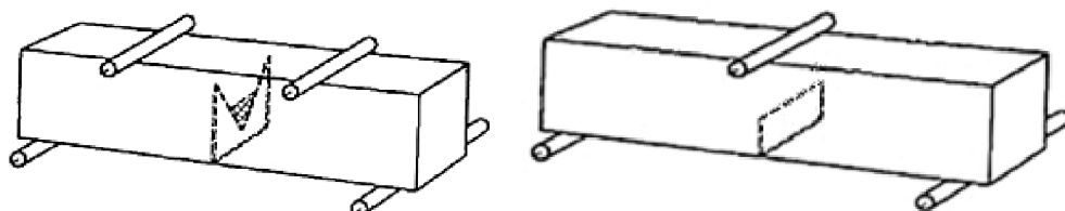
Obr. 2.15: Čtyřbodový ohyb-vzorek s vrubem typu chevron (vlevo) a třibodový ohyb-vzorek s rovným vrubem
