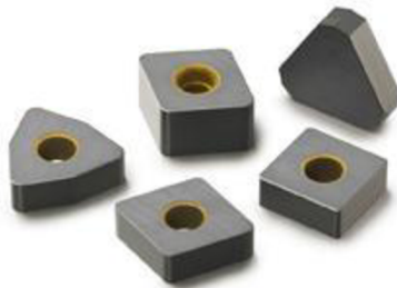
Obr. 2.2: Řezné destičky ze Sialonu [3]
