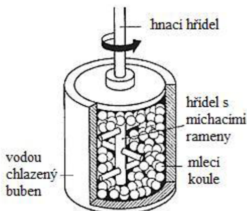
Obr. 2.6: Schéma atritoru [8]
