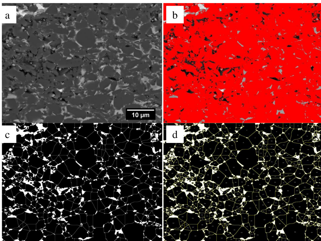
Obr. 4.5: a) původní snímek, b) naprahovaný snímek, c) zrna separovaná ze struktury s doplněnými hranicemi zrn, d) zanalyzovaný snímek s očíslovanými zrnky, zvětšení 3000x
