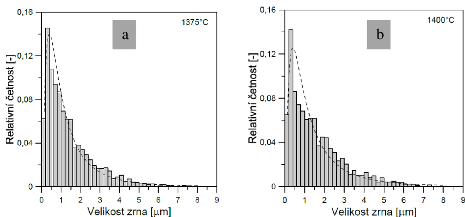
Obr. 5.17: Distribuce velikosti zrn TiB 2 ve vzorku slinutém a) při 1375 °C, b) při 1400 °C
