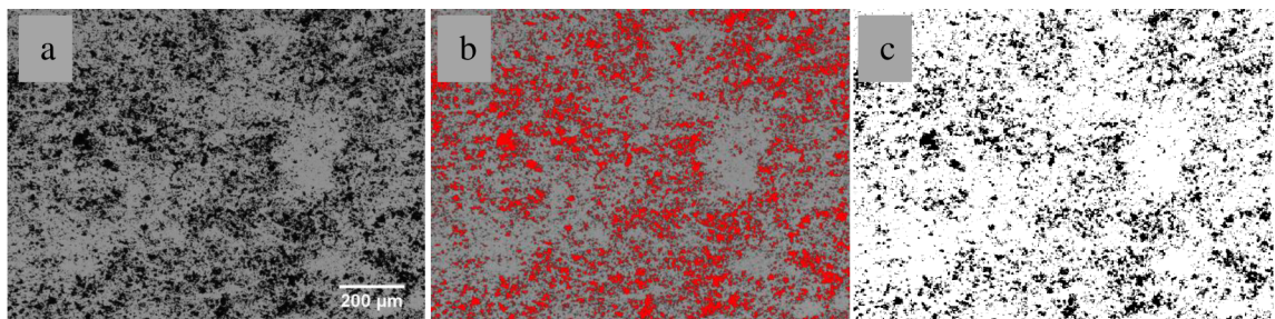
Obr. 5.12: Analýza množství pórů, slinování při 1300 °C a) původní fotografie, b) naprahovaná fotografie, c) upravená fotografie pórů separovaných ze struktury, zvětšení 240x
