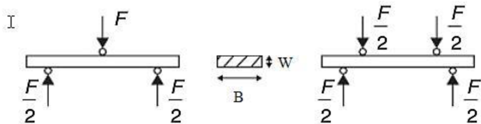
Obr. 2.14: Schéma zatěžování vzorku při zkoušce třibodovým respektive čtyřbodovým ohybem, kde F je působící síla, B a W rozměry průřezu vzorku [21]
