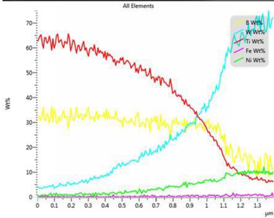
Obr. 5.34: Liniová chemická analýza přechodu ze zrna \text{TiB}_2 do slitiny NiW
