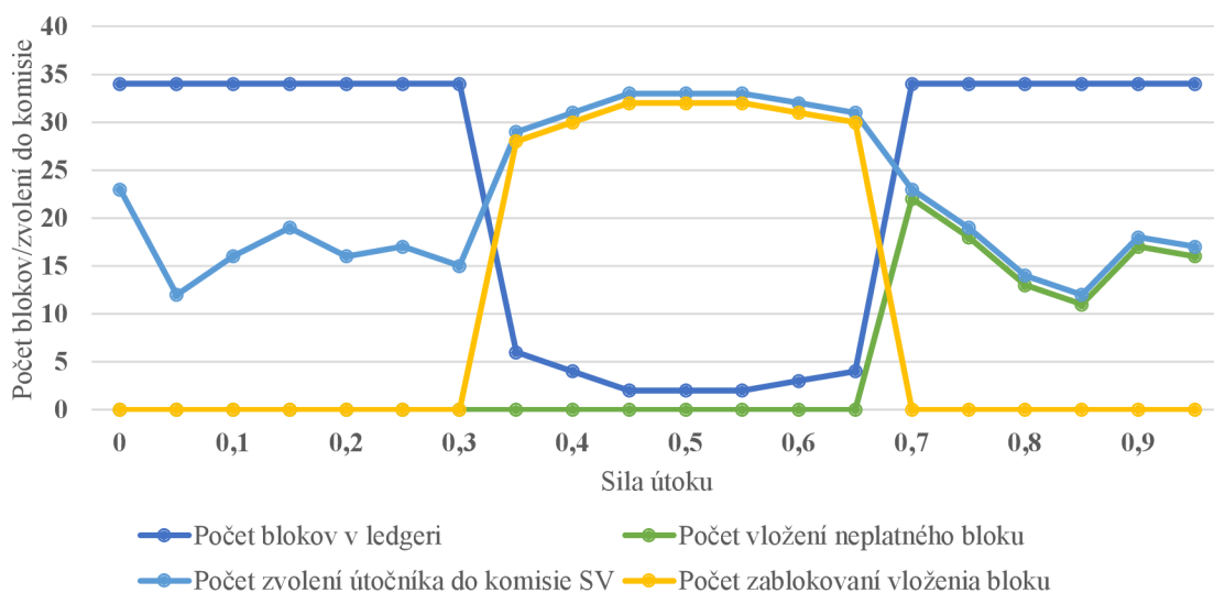
Obr. 6.10: Vplyv sily útoku na počet úspešných vložení neplatných blokov útočníkom, či zablokovaní vloženia platných blokov do ledgera pri pevne danej veľkosti stávky čestných voličov. Graf zobrazuje aj počet zvolení útočníka do komisie vo fáze Soft vote.
