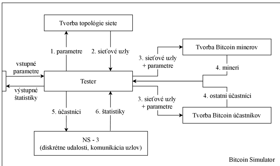
Obr. 5.1: Schéma nástroja Bitcoin Simulator zobrazujúca jednotlivé moduly a zjednodušený proces simulácie.
