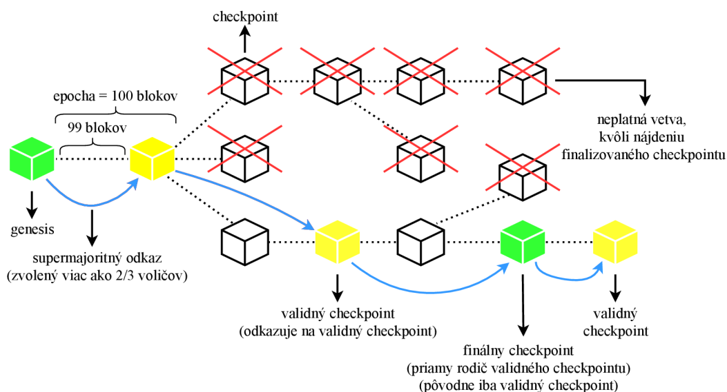
Obr. 3.3: Strom kontrolných bodov obsahujúci blok genesis (prvý validný finálny checkpoint), validné body (žlté), finálne body (zelené) a supermajoritné odkazy (modré). Bodkované čiary medzi kontrolnými bodmi predstavujú 99 blokov vytvorených PoW algoritmom. Po nájdení finálneho checkpointu sa ostatné vetvy považujú za neplatné [16, 62].
