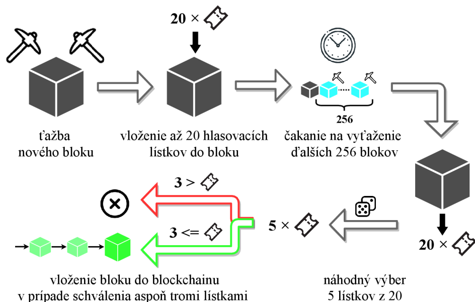
Obr. 3.10: Priebeh schvaľovania vytáženého bloku proof-of-stake voličmi [53].
