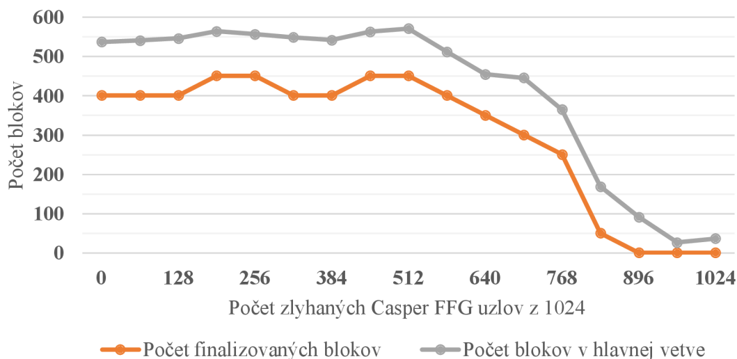
Obr. 6.6: Vplyv počtu zlyhaných Casper FFG uzlov na finalizáciu blokov. Simulácia 5000 minút protokolu Casper FFG so základným protokolom Bitcoin s blokmi pevnej veľkosti 500 KB. Počet Bitcoin minerov bol pri každej simulácii 64 a počet Casper FFG validátorov bol 1024.
