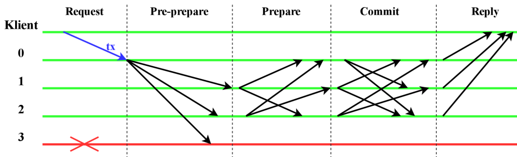
Obr. 3.1: Priebeh PBFT operácie skladajúca sa z fáz: request, pre-prepare, prepare, commit, reply. Uzol 0 predstavuje primárny uzol, uzly 1 až 3 sú repliky. U repliky číslo 3 došlo k výpadku. [21]
