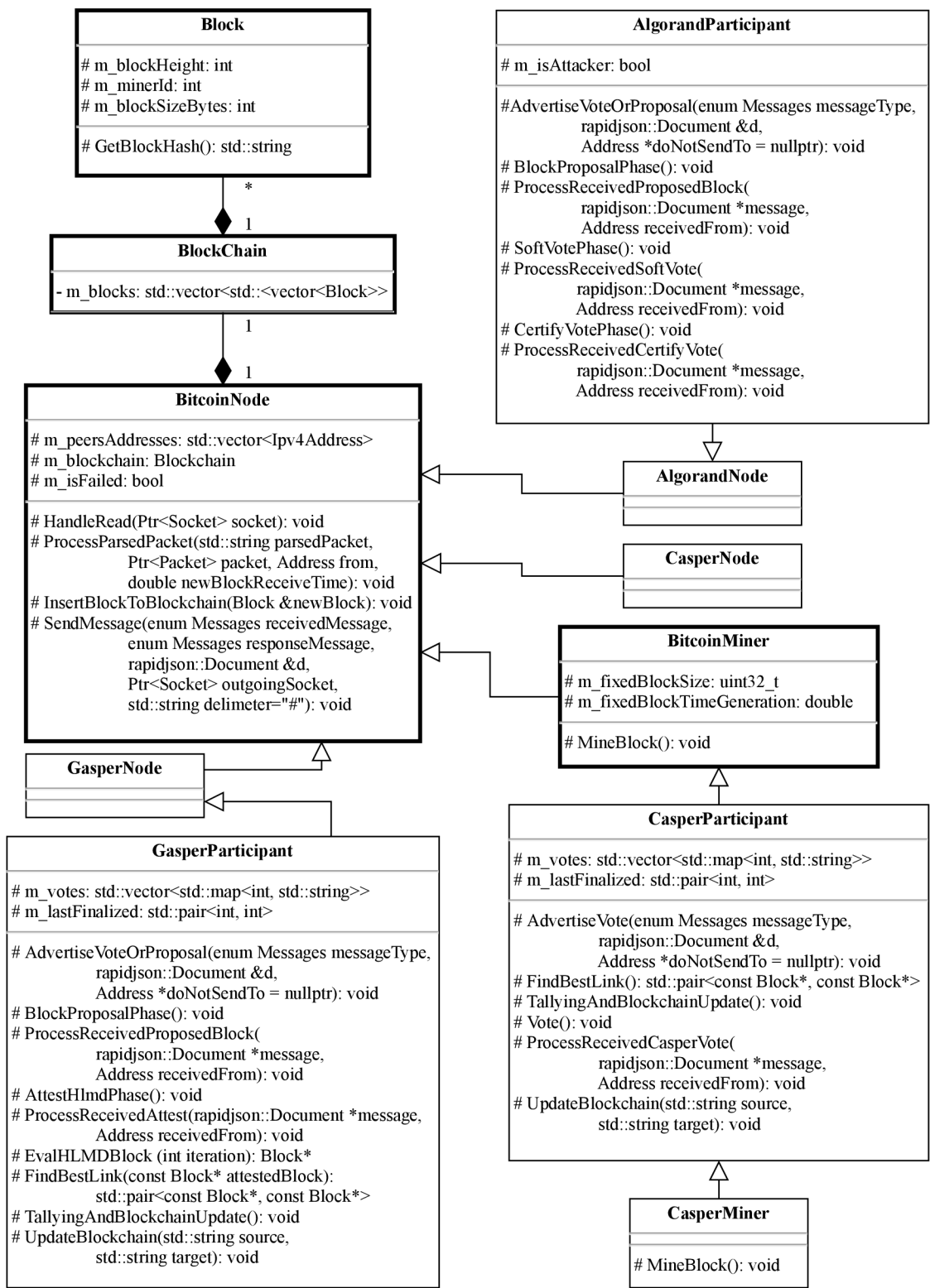
Obr. A.2: Diagram tried slúžiacich pre simuláciu protokolov Algorand, Casper FFG a Gasper. Hrube zvýraznené sú pôvodné triedy nástroja Bitcoin Simulator. V diagrame sú zaznamenané iba najdôležitejšie vlastnosti a metódy tried.
