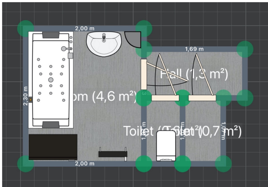
Obrázek 7 Nynější dispozice koupelny
