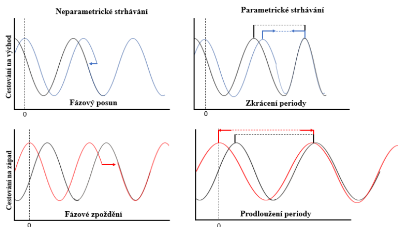
Obrázek 18: Modely normalizace cirkadiálních rytmů enviromentálním prostředím. V „neparаметrickém“ modelu je normalizace dosáhnuta fázovým posunem, který způsobují podněty enviromentálního prostředí (cyklus světla a tmy). Na druhé straně „parametrický“ model se soustředí na rychlost pohybu cirkadiálních hodin, a normalizace se dosahuje modulací volně běžící periody. Na základě toho se předpokládá, že sloučeniny, které zvyšují velikost fázového posunu snižují pásmovou nemoc prostřednictvím neparаметrického mechanismu, zatímco sloučeniny ke zkrácení a prodloužení periody snižují pásmovou nemoc zrychlením nebo zpomalením hodin, čímž se zrychluje opětovná normalizace při cestování na východ, respektive na západ (Tamai et al., 2018).
