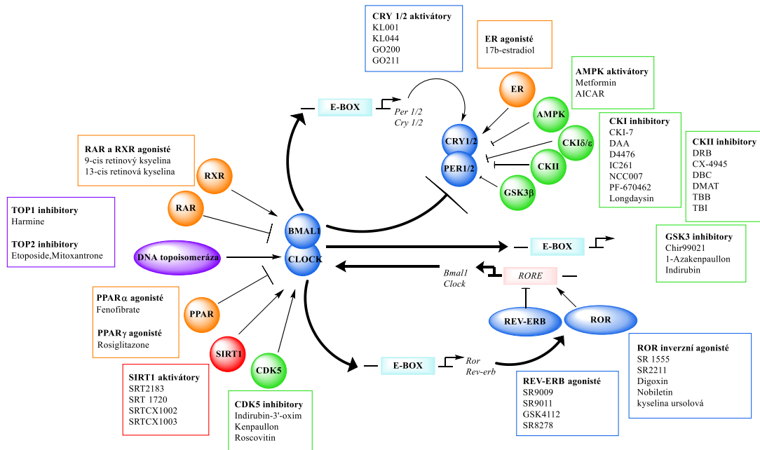
Obrázek 7: Model jednotlivých TTFL společně se zástupci jejich klíčových modulátorů. Modře proteiny hodinového jádra, zeleně regulační kinázy, oranžově ostatní jaderné receptory, červeně SIRT1 modulátory, fialově DNA topoizomerázy. Základní komponenty TTFL představují CLOCK:BMAL1, PER:CRY a ROR/REV-ERV, jejichž modulací dochází ke změnám cirkadiální amplitudy, fáze a periody. AMPK (5'AMP-aktivovaná proteinkináza), AR (androgenní receptory), CDK5 (cyklindependentní kináza 5), CKI kaseinkináza 1), CKII (kaseinkináza 2), CRY1/2 (krytochrom 1/2), GSK3 (glykogensyntázakináza 3), PPAR (receptory aktivované peroxizomovými proliferátory), RAR (receptory kyseliny retinové), REV-ERB (retinoic acid-related orphan receptor), ROR (retinoic acid-related orphan receptor), RXR (retinoid X receptory), SIRT 1(silent information regulator 1) (He a Chen, 2016).
