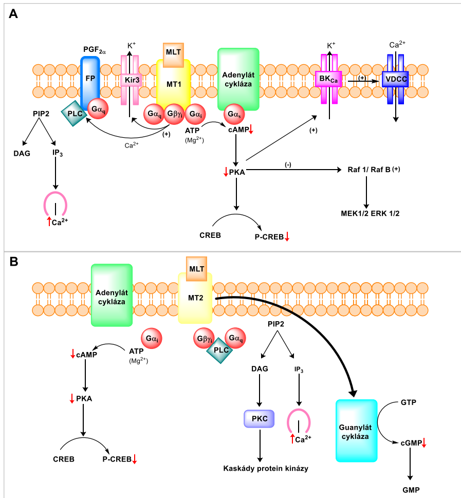
Obrázek 4: Signální dráhy aktivované prostřednictvím MT1 a MT2 receptorů. A Signální dráhy po aktivaci receptoru MT1 spojené s G proteiny Gα i a Gα q . B Signální dráha spojená s aktivací receptoru MT2. ATP (adenosintrifosfát), BK Ca (vápníkem aktivovaný draslíkový kanál), cAMP (cyklický adenosinmonofosfát), cGMP (cyklický guanosinmonofosfát), CREB (cAMP-responsive element binding protein), DAG (1,2-diacylglycerol), FP (receptor pro prostaglandin F 2α ), Ga (G-proteiny), GMP (guanosinmonofosfát), GTP (guanosintrifosfát), IP 3 (inositol-1,4,5-trifosfát), Kir3 (draselný kanál spřažený s G proteinem), MEK1/MEK2 (mitogenem aktivovaná proteinkináza kináza; EC 2.7.12.2), MLT (melatonin), PKA (proteinkináza A; EC 2.7.11.11), P-CREB (fosforylovaný CREB), PIP 2 (fosfatidylinositol-4,5-bisfosfát), PGF 2α (prostaglandin F 2α ), PKC (proteinkináza C; EC 2.7.11.13), PLC (fosfolipáza C; EC 3.1.4.3), Raf 1/Raf B (proto-onkogen serin/threonin proteinkináza; EC 2.7.11.1), VDCC (na napětí závislý Ca 2+ kanál). (Upraveno podle Masana a Dubocovich, 2001).
