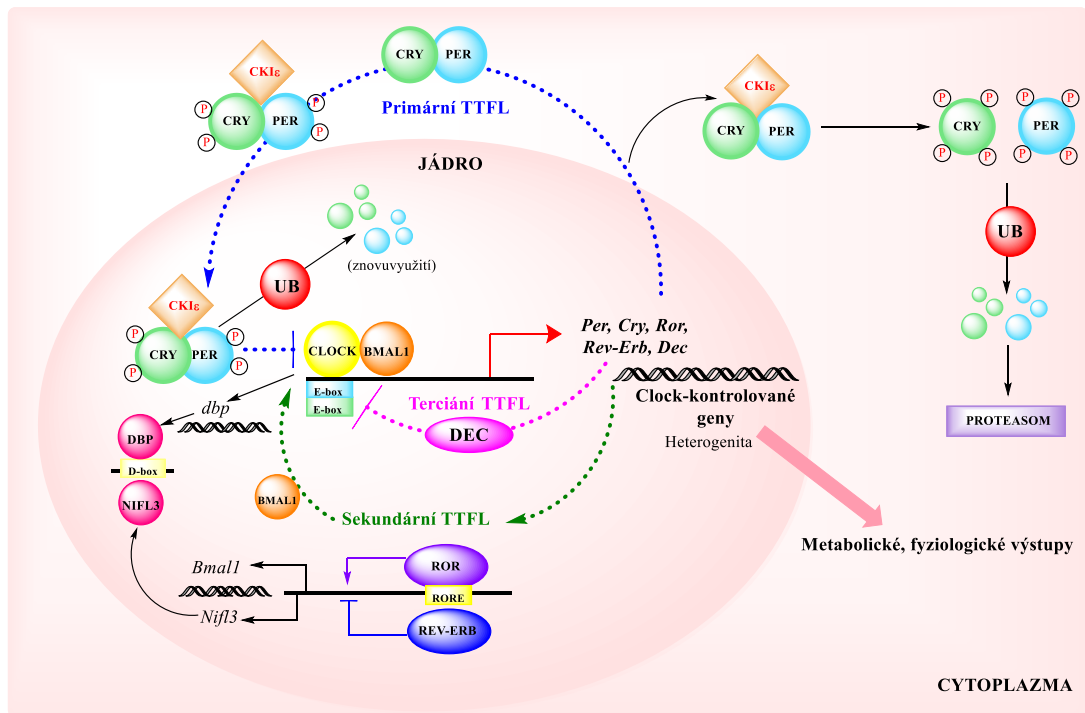
Obrázek 6: Model molekulární cirkadiánní oscilace centrální TTFL u savců: Model znázorňující tři základní oscilační smyčky cirkadiánního rytmu. Primární, zahrnující vznik komplexu CRY:PER a jeho následnou fosforylaci skrze CKIε a translokaci do jádra, kde interagují s komplexem CLOCK:BMAL1, což vede k inhibici transkripce v průběhu noci. Sekundární smyčka představuje zapojení transkripčních faktorů ROR a REV-ERBs, které mají funkci transkripčních aktivátorů a represorů rytmického řízení transkripce BMAL1. Terciální smyčka představuje transkripční represory DEC, které inhibují transkripci indukovanou komplexem CLOCK:BMAL1 kompeticí při vazbě na E-box regulační sekvence genů. BMAL1 (Brain muscle arnt like 1), CKIε (kaseinkináza ε; EC:2.7.11.1), CLOCK (circadian locomotor output cycles kaput), CRY (krytochrom), DBP (albumin side D-binding protein), NIFL3 (Nuclear factor Interleukin 3 regulated), P (fosfát), PER (period), ROR (retinoic acid-related orphan receptor), TTFL (transkripčně-translační zpětnovazebná smyčka), UB (ubikvitinace) (Upraveno podle Ki et al., 2015).
