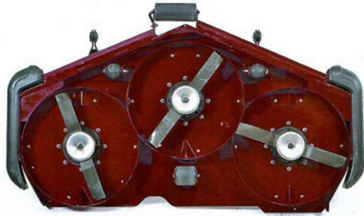
Obrázek 6 Kosící ústrojí rotační sekačky (Hrabě et al. 2009)
