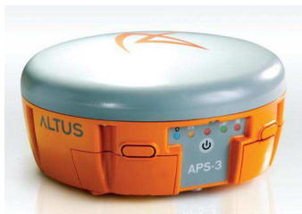
Obrázek 15 – foto - Aparatura GPS Altus [16]
