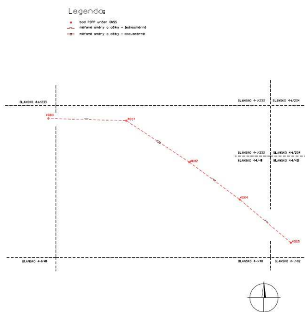
Obrázek 17 - Přehledný náčrt měřické sítě Vilémovice [15]
