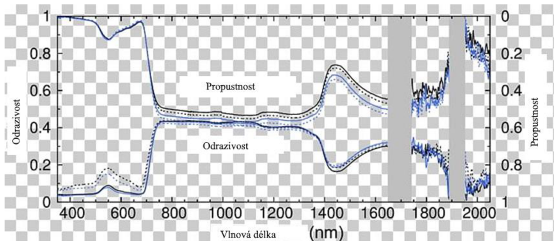
Obrázek 4.2 – Transmitta a reflektance (Dvořáková, 2016)
