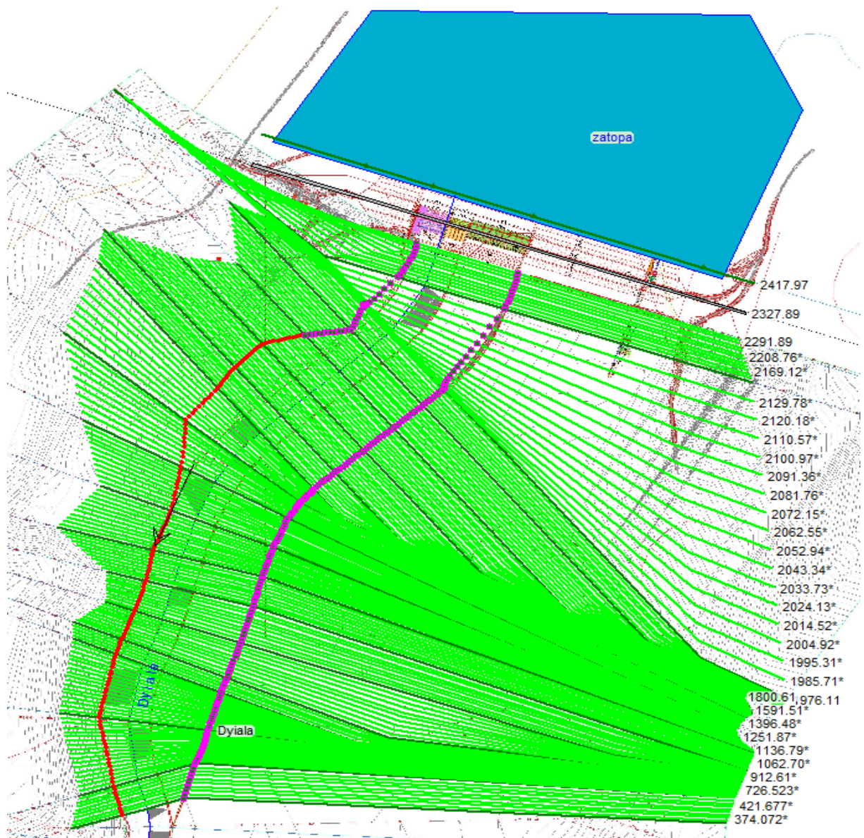
Obr. 3.5 Situace geometrických dat daného úseku v programu HEC - RAS
