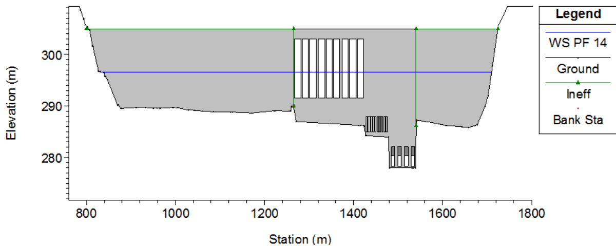
Obr. 3.22 Umístění inefektivních ploch v podélném řezu hrázi (WS – hladina vody v profilu, Ground – terén, Ineff – inefektivní plocha, Bank Sta – břehová čára, Elevation – nadmořská výška, Station – staničení)
