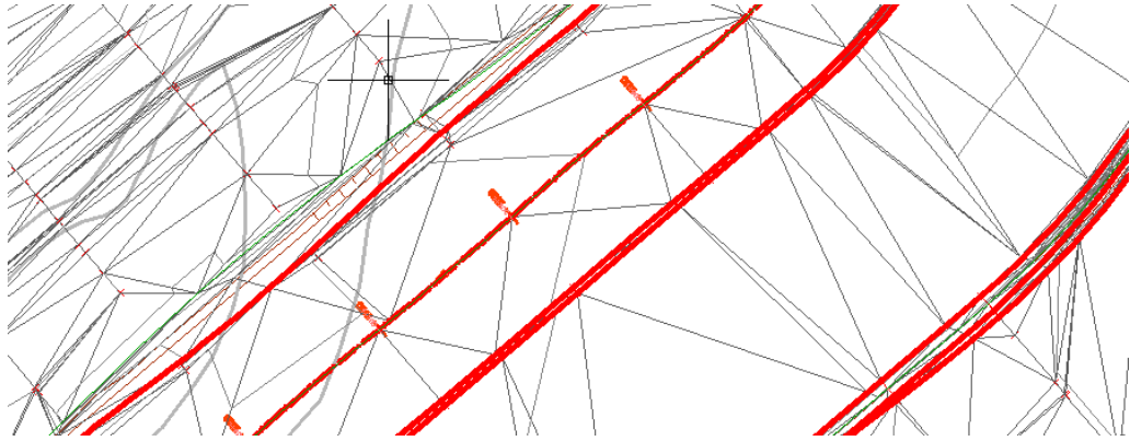
Obr. 3.1 Výřez z povrchu TIN s povinnými spojnicemi
