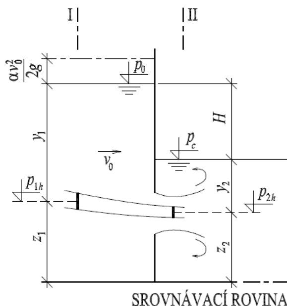
Obr. 3.17 Schéma výtoku ponořeným otvorem ve svislé stěně [3]
