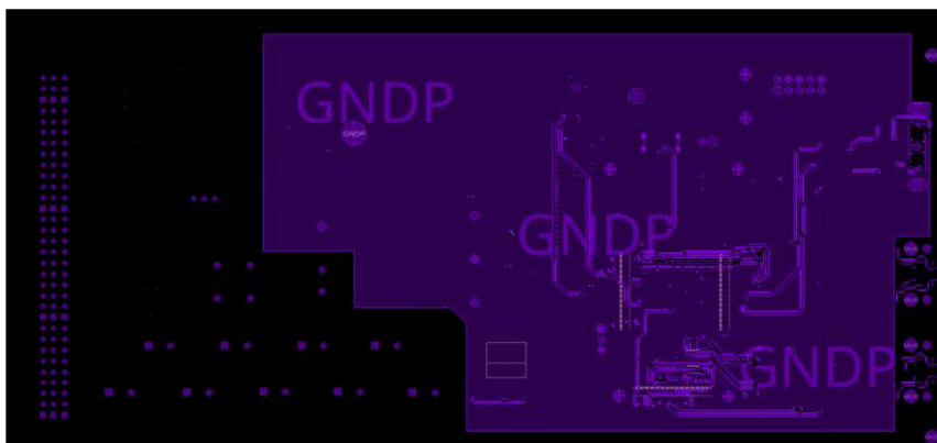
Obrázek 59 - Nerovnoměrné zatížení desky - Špatné řešení
