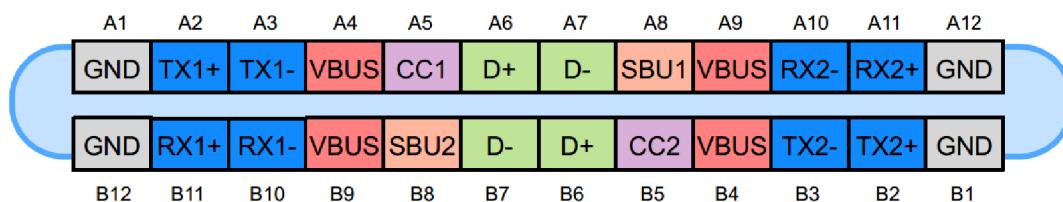
Obrázek 28 - Kontakty pro konektor USB-C [19]
