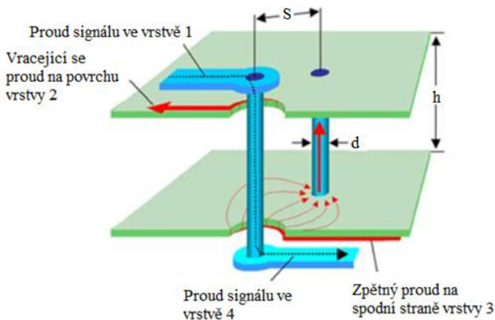
Obrázek 67 - Realizace ethernetového portu na DPS [51]
