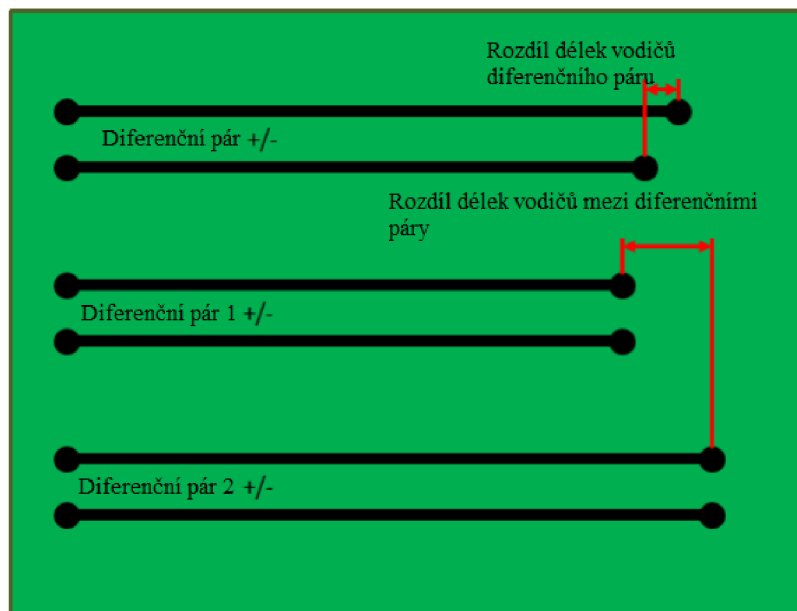
Obrázek 52 - Různé délky vodičů diferenčního páru [46]
