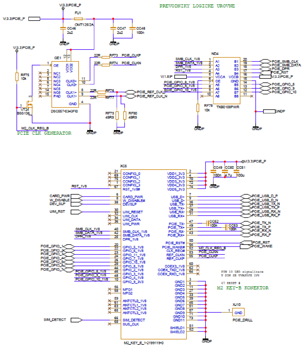
Obrázek 91 - Schéma PCIe konektoru
