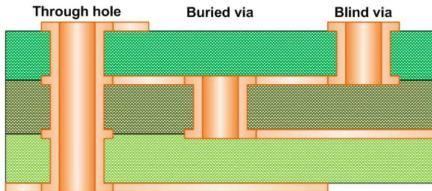
Obrázek 57 - Znáornění rozdílu mezi Via, blind via a burried via [45]
