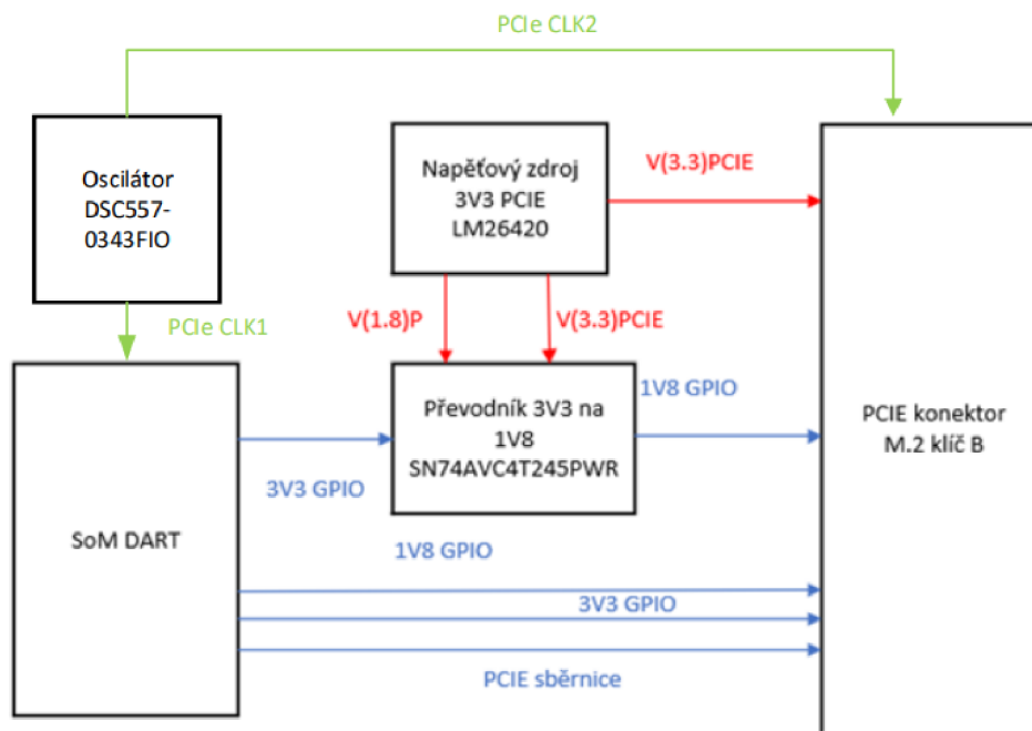
Obrázek 44 - Blokové schéma PCIe sběrnice
