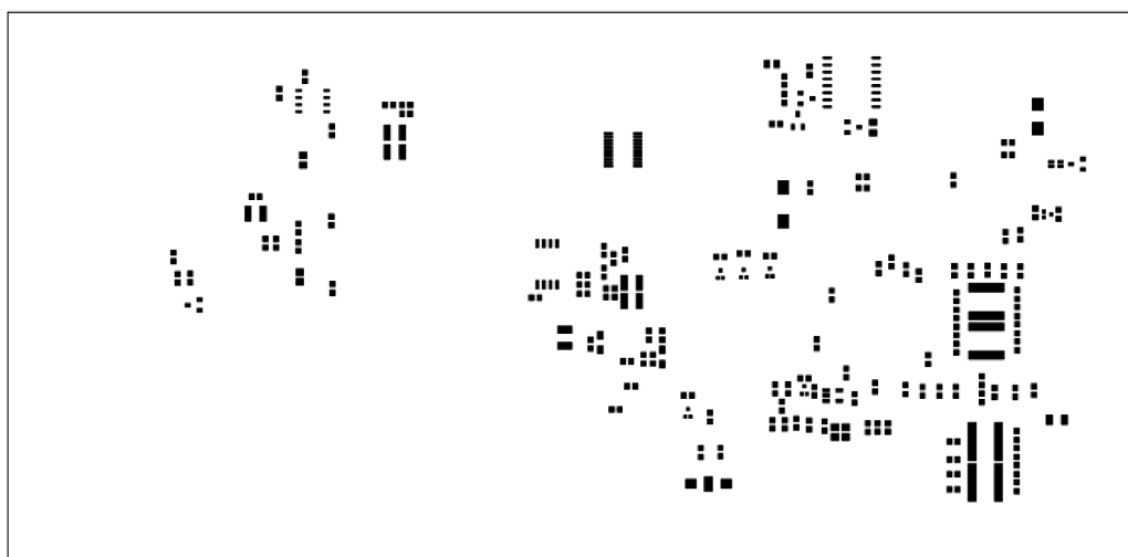
obrázku 76 - Vzor pro nanesení pájecí pasty pro vrstvu BOT
