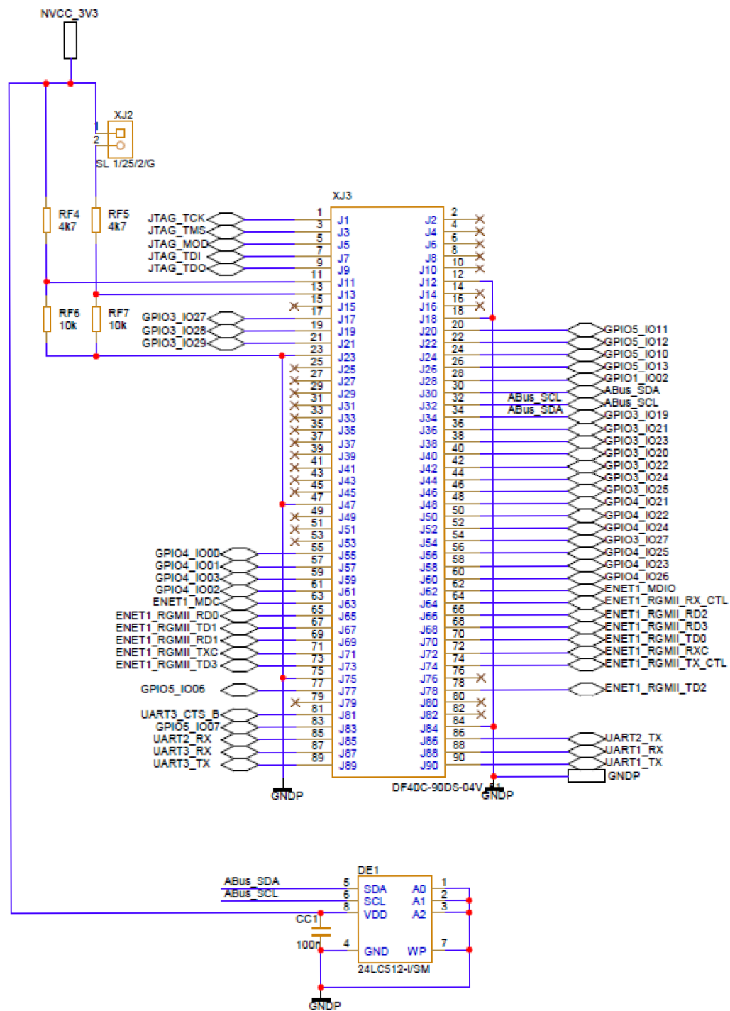
Obrazek 85 - schéma konektoru 2 SoM DART
