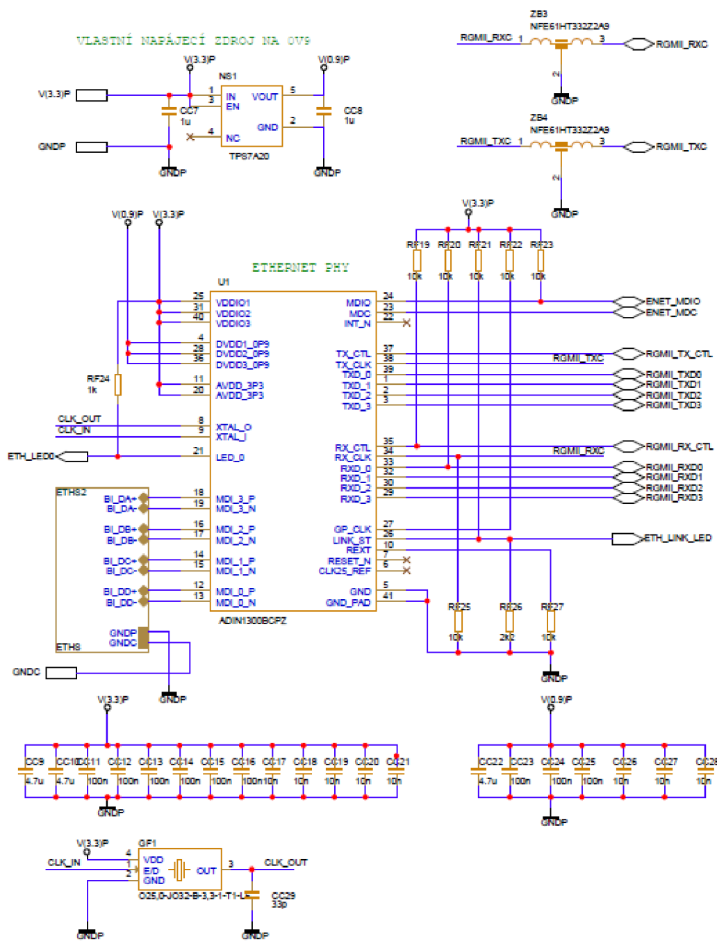
Obrázek 88 - Schéma fyzikální vrstvy ethernetu
