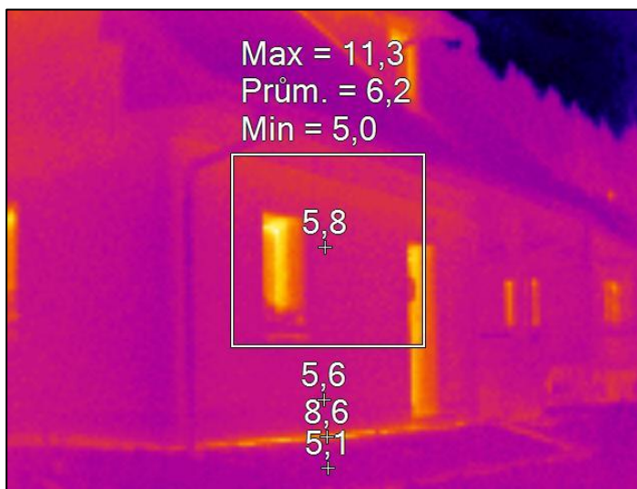
LINEÁRNÍ TEPELNÝ MOST U ZÁKLADŮ
