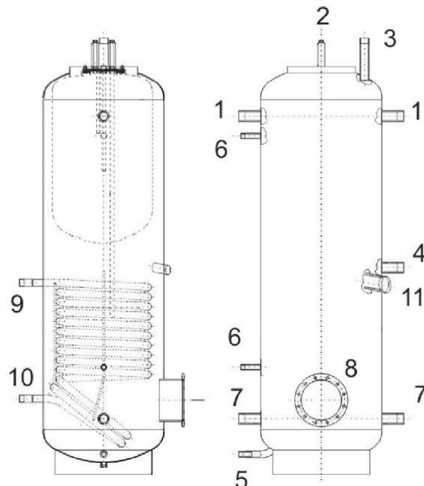
Obrázek 25 - AKUMULAČNÍ NÁDRŽ DRAŽICE
