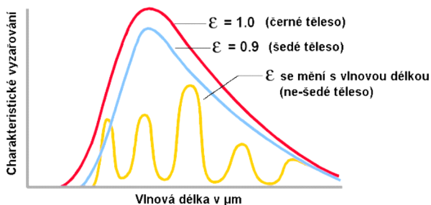
Obrázek 8 - EMISIVITA TĚLES
