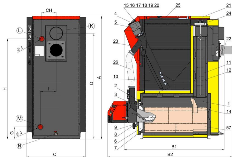
Obrázek 24 - KOTEL ATMOS D15PX
