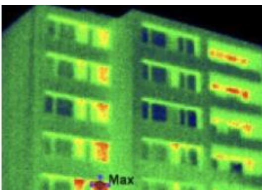
Obrázek 16 - TERMOGRAFIE BUDOV
