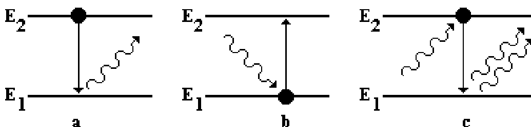
Obrázek 11 - ABSORPCE
