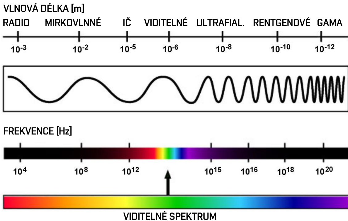
Obrázek 4 - ELEKTROMAGNETICKÉ SPEKTRUM
