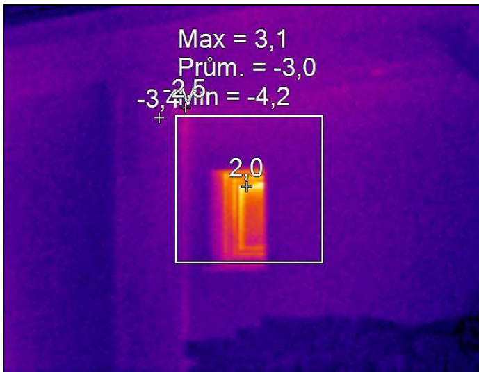
BODOVÝ TEPELNÝ MOST V ROHU
