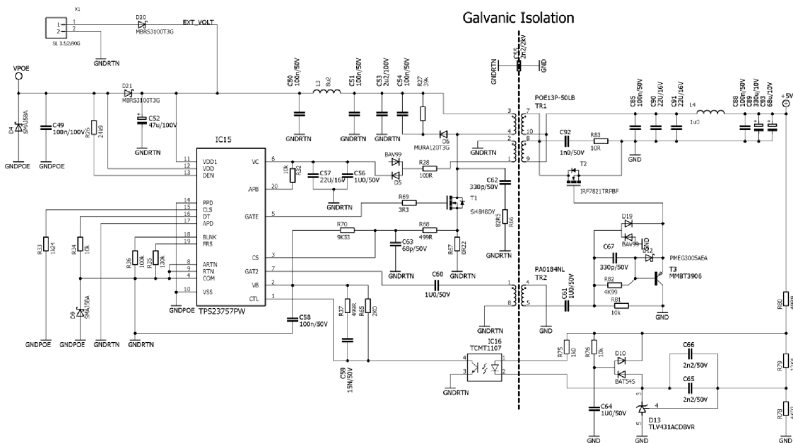
Obrázek 13: Zapojení TPS23757
