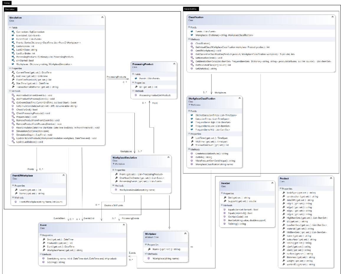
Obrázek 6.5: Diagram tříd balíčku Mining.
