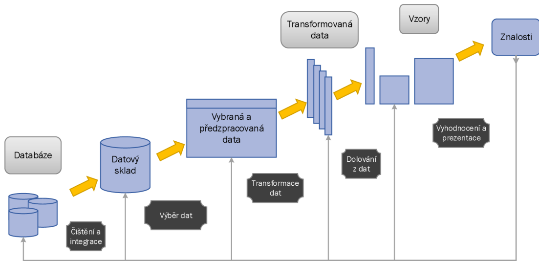
Obrázek 2.1: Schéma procesu získávání znalostí z databází, převzato a upraveno z webu [12]
