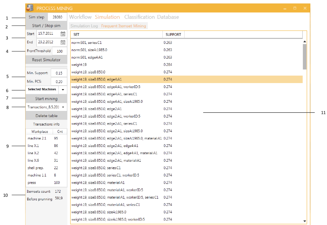
Obrázek A.1: Ukázka hlavního okna aplikace se simulátorem.
