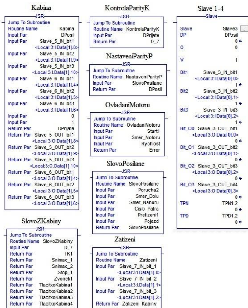
Obrázek 6.2 Vstupní a výstupní proměnné rutin a funkcí
