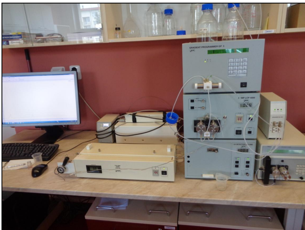
Obr. 62: Kapalinový chromatograf - stanovení vitamínu C
