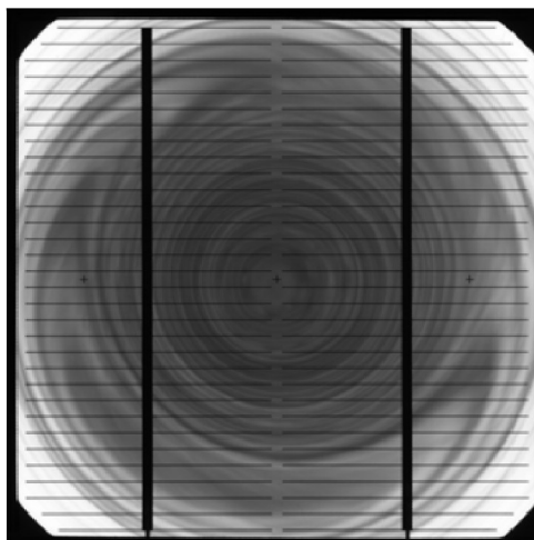
Obr. 3.2: Vírový defekt [10]
