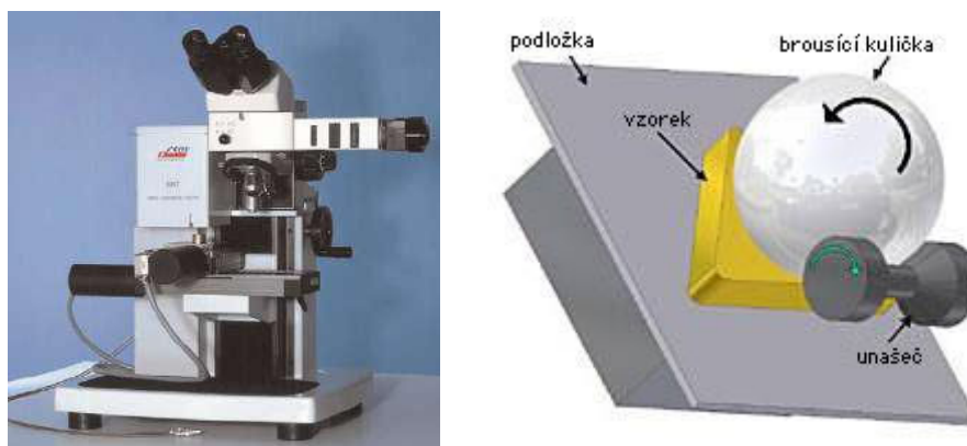
Obr. 1.50 Nanoindentor a schéma kalotestru 34, 45
