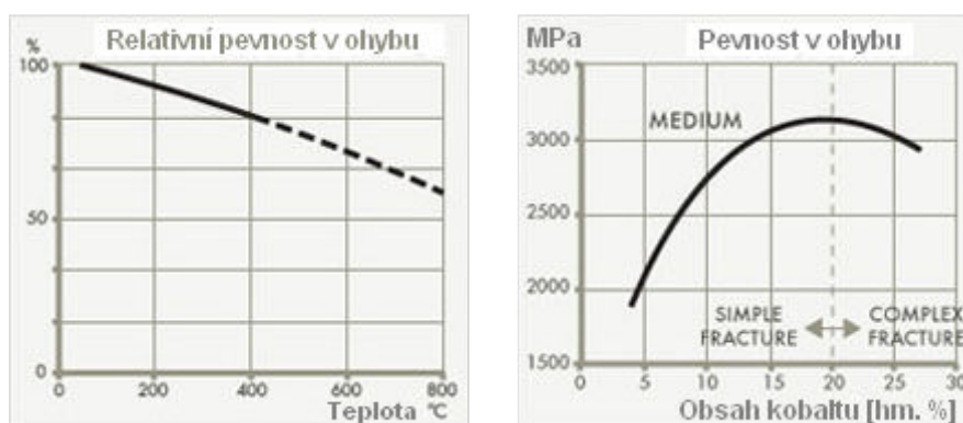
Obr. 1.46 Závislost relativní pevnosti v ohybu na teplotě a závislost pevnosti v ohybu na hmotnostním procentu obsahu kobaltu 40
