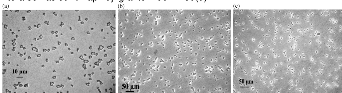
Obr. 1.40 Plocha substrátu po depozici povlaku TiN a po odstranění keramických korálek pomocí ultrazvukových vibrací. Příklady použití různých velikostí korálek (a) 1,5 µm, (b) 5 µm, (c) 10 µm 52
