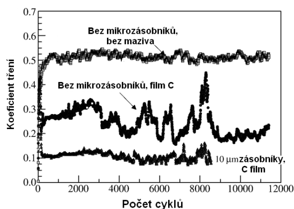
Obr. 1.42 Výsledky testu Pin – on – Disc za použití vrstvy amorfniho uhlíku jako tuhého maziva 52
