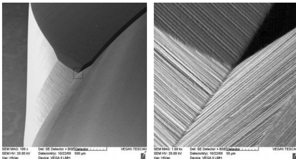
Obr. 1.31 Povrch nástroje s povlakem Darwin 20
