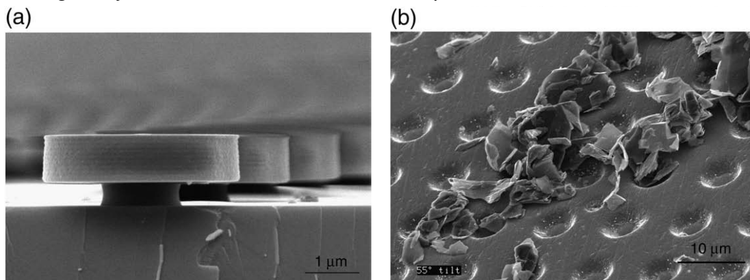
Obr. 1.38 a) Fotorezistentní ostrůvky na substrátu b) Povrch po povlakování, utváření děr a aplikaci grafitu 18
