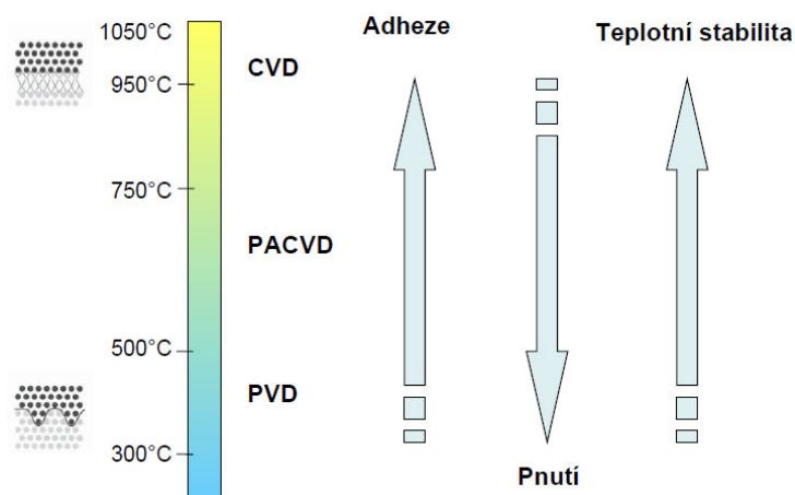
Obr. 1.30 Porovnání vlastností vrstvy při různé teplotě (metodě) povlakování 34
