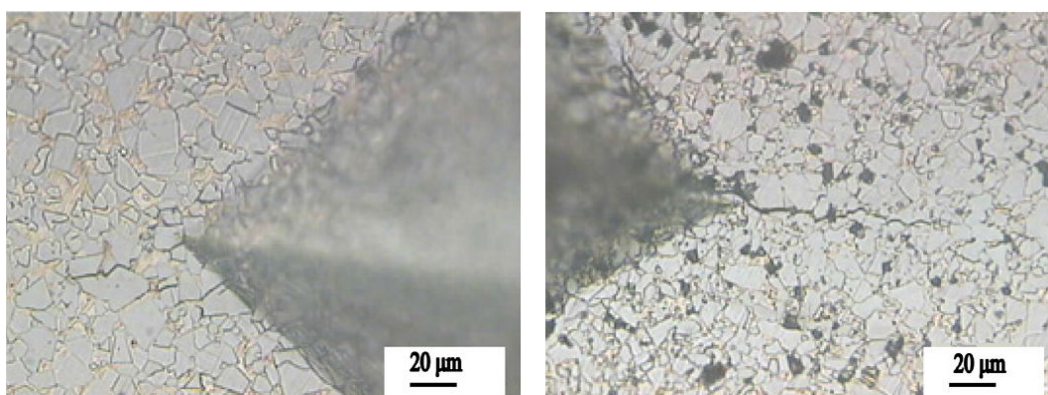
Obr. 1.11 Šíření trhliny, v rozích otisku, po zkoušce mikrotvrdomi podle Vickerse, ve vnější vrstvě s dvoufázovou strukturou a v tvrdém jádru slinutého karbidu s trojfázovou strukturou 51
