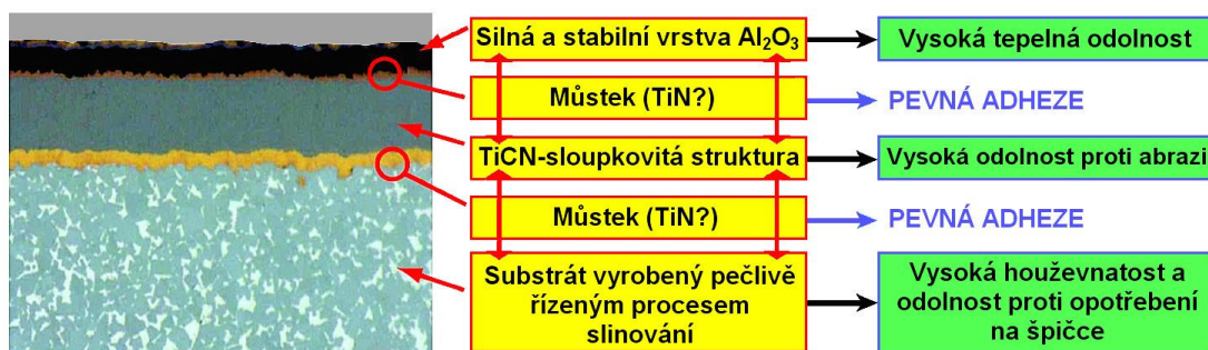
Obr. 1.21 Povlak 3. generace od firmy Toshiba 21
