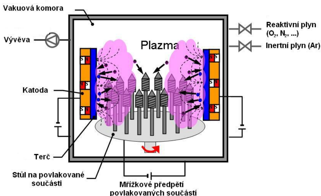
Obr. 1.26 Schéma komory pro magnetronové napařování 3
