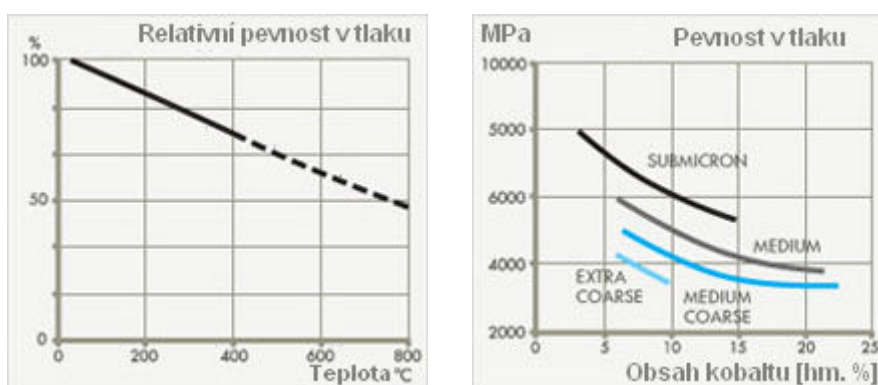
Obr. 1.47 Závislost relativní pevnosti v tlaku na teplotě a závislost pevnosti v tlaku na hmotnostním procentu obsahu kobaltu, pro rozdílné zrnitosti slinutých karbidů viz. tab. 1.4 40
