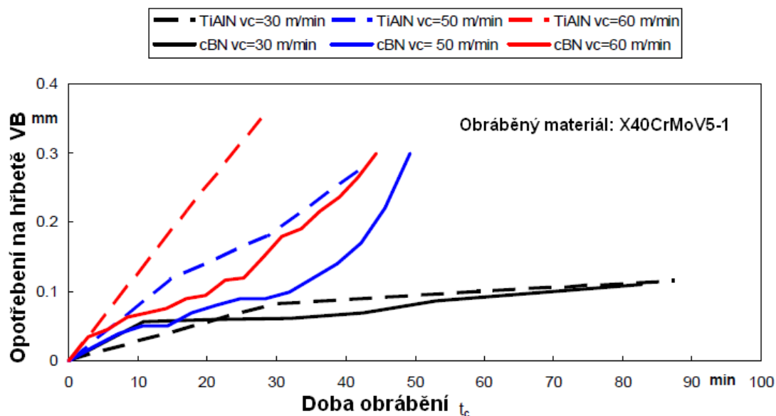
Obr. 1.34 Závislost opotřebení VB na času obrábění standardních povlakovaných řezných destiček a destiček deponovaných vrstvou KNB 4
