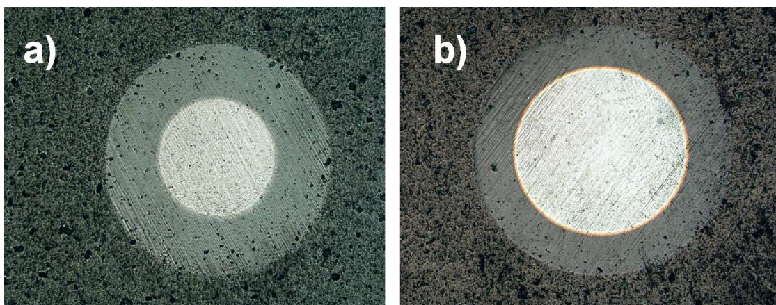
Obr. 1.20 Kalotest povlaků 34 :
