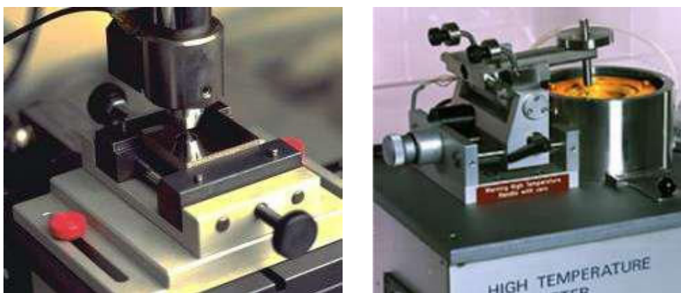
Obr. 1.51 Scratch tester a zařízení pro provádění testů „PIC – on – DISC“ (tribometr) 34
