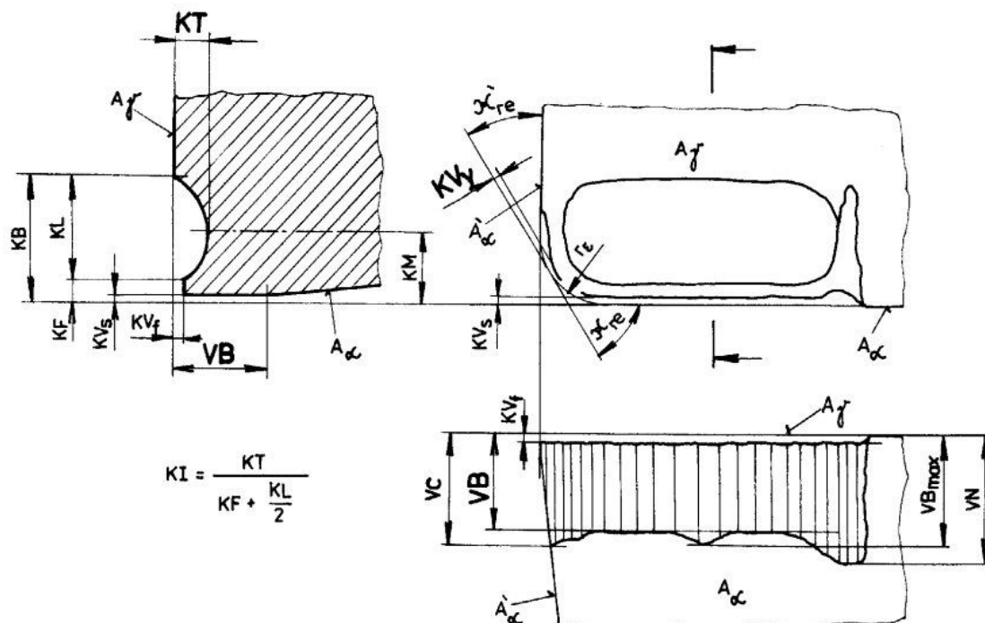
Obr. 3.2 Kritéria opotřebení řezného nástroje 25
