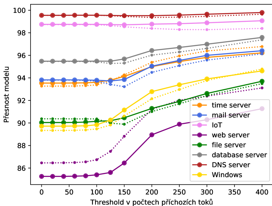
Obrázek C.3: Přehled přesnosti jednotlivých klasifikátorů při aplikaci určitého thresholdu v počtu příchozích toků . Plná čára klasifikátoru představuje celkovou přesnost modelu, přerušovaná čára zobrazuje metriku F1-score predikovaného štítku (typu zařízení).
