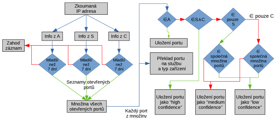
Obrázek 5.1: Způsob přidělení štítků o dostupných službách na zařízení a typu zařízení. Znak A reprezentuje službu ADiCT, znak S reprezentuje službu Shodan a znak C reprezentuje službu Censys. Pokud je určitá podmínka (modré kosočtverce) splněna, proces pokračuje po zelené šipce. Pokud podmínka splněna není, pokračuje se po šipce červené. Nejprve dojde ke kontrole, zda jsou informace ze systémů ADiCT, Censys a Shodan aktuální. Pokud ano, seznamy portů se sjednotí a zkoumá se, v jakých službách se daný port vyskytuje. Společná množina portů je rovna sjednocení portů, které skenují na zařízeních zároveň obě služby Shodan i Censys.
