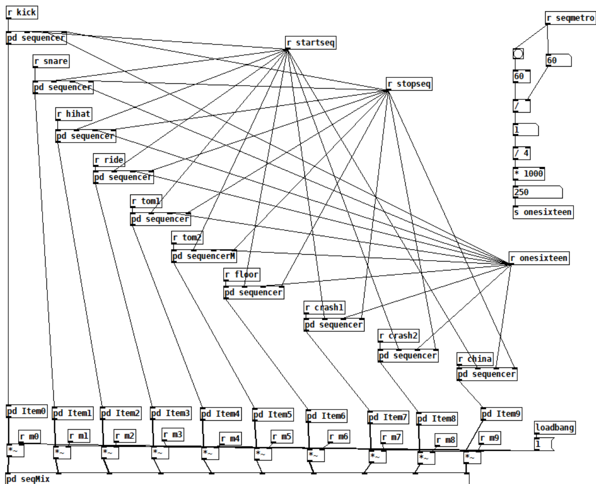
Obr. 4.18: Sekvencer
