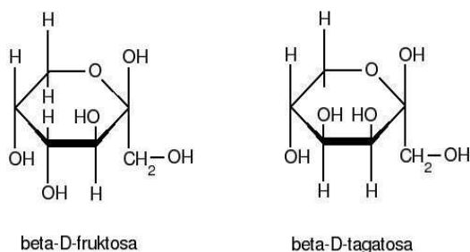
Obrázek 1 Porovnání struktury \beta -D-fruktosy a \beta -D-tagatosy
