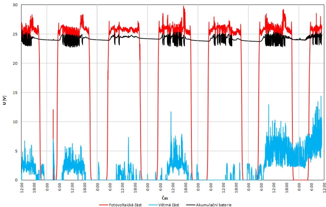
Obr. 7-1 Časový průběh napětí
