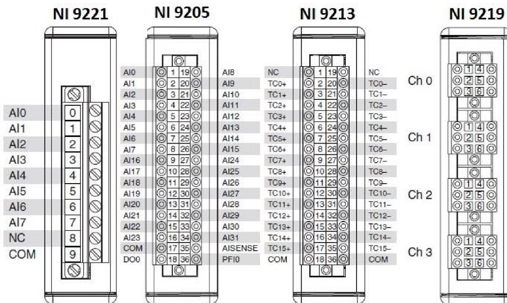
Obr. 6-4 Označení vstupů měřicích karet [39]
