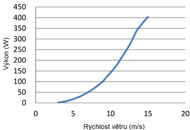
Obr. 4-6 Výkonová charakteristika větrné elektrárny [34]
