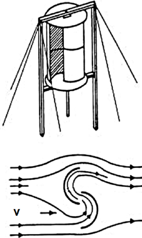
Obr. 3-3 Savoniův motor
