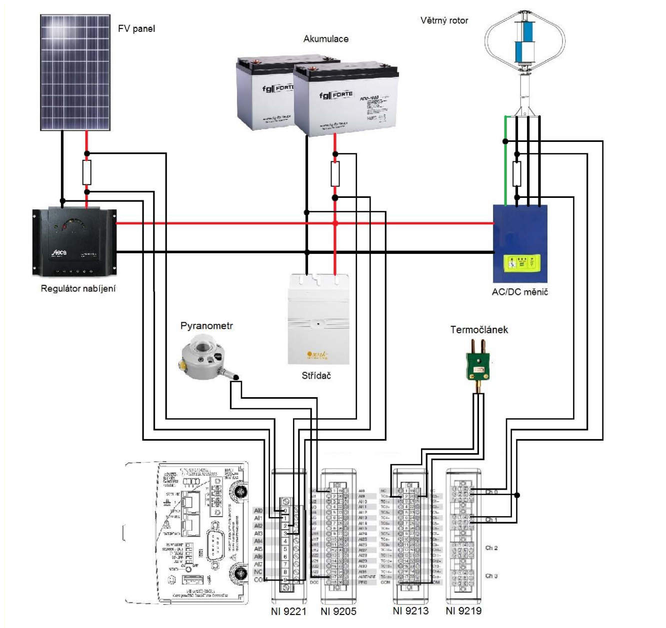
Obr. 6-3 Zapojení měřicího systému
