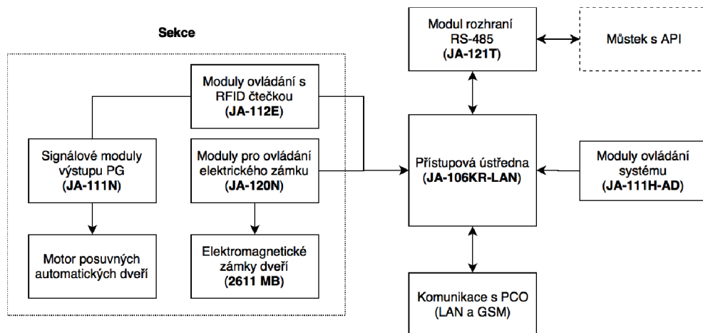
Obrázek 4.3: Schéma přístupového systému
