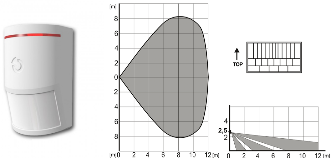
Obrázek 3.6: Sběrníkový PIR detektor pohybu - JA-110P [3]
