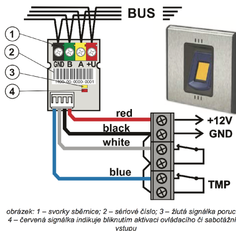
Obrázek 3.14: Sběrnice modul ovládání systému - JA-111H-AD [3]
