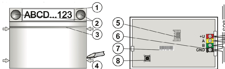
Obrázek č. 1: 1 – ovládací segment; 2 – tlačítka segmentu; 3 – prosvětlené aktivační tlačítko s RFID čtečkou; 4 – západky pro otevření modulu;
