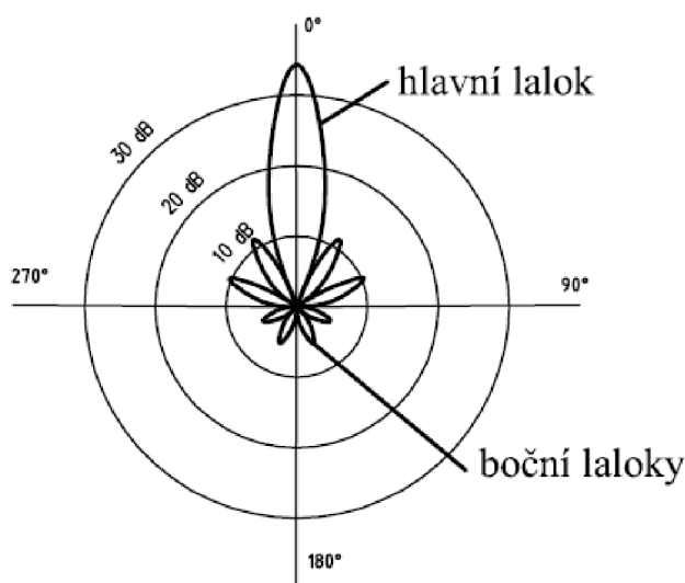
Obr. 1.1 Typický horizontální vyzařovací diagram směrové antény primárního radaru [12]
