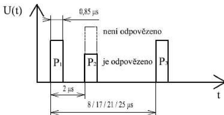
Obr. 2.4 Dotaz SSR [12]
