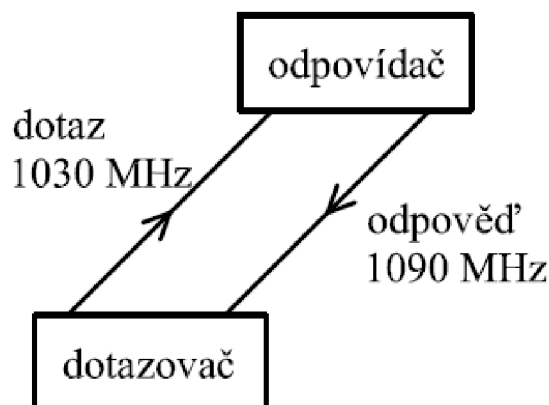
Obr. 2.3 Dotaz–odpověď [12]
