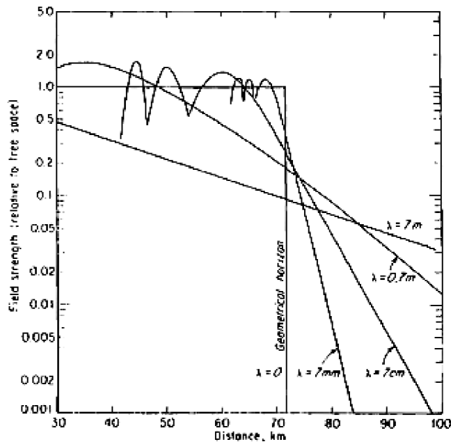
Obr. A-7 Radarový horizont [23]
