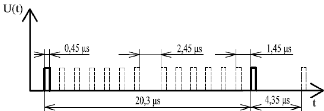
Obr 2.5 Odpověď SSR [12]
