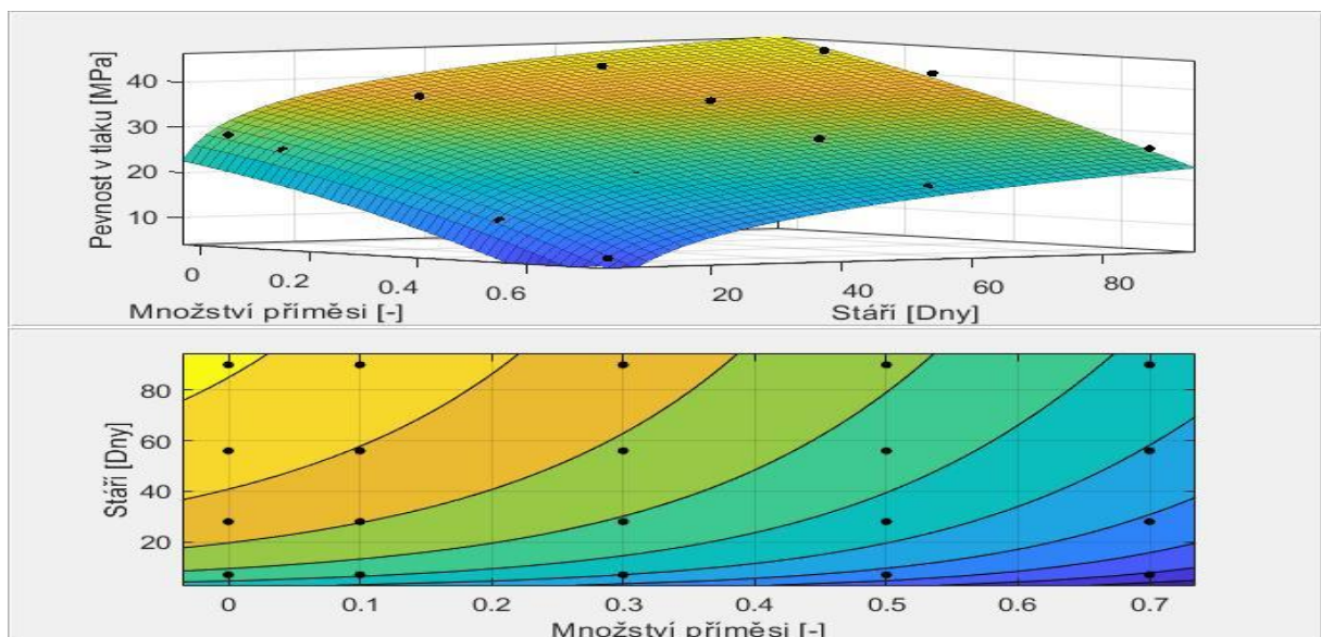
Obrázek 17: Grafické znázornění funkce pevnosti v tlaku pro popílek Opatovice
