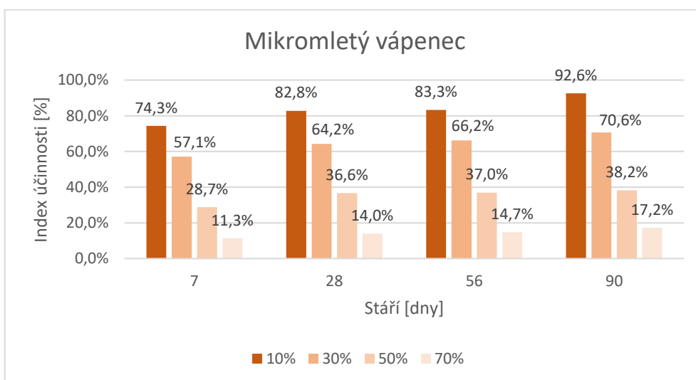
Graf 15: Index účinnosti pro mikromletý vápenec
