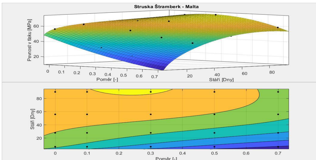
Obrázek 12: Grafické znázornění funkce pevnosti pro strusku Štramberk
