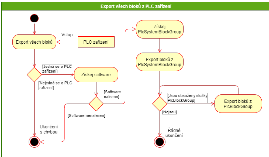
Obr. 5.5: Aktivita diagram - Exportování všech bloků
