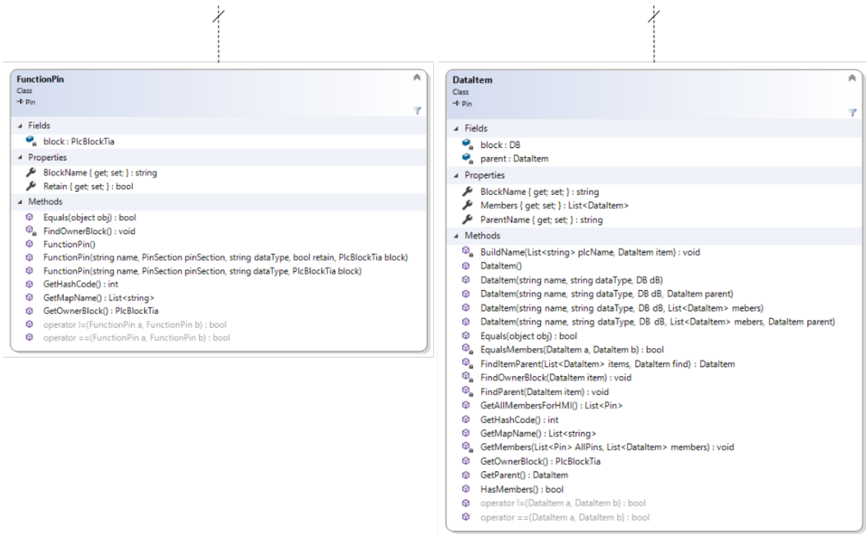
Obr. A.6: Class diagram 6. část
