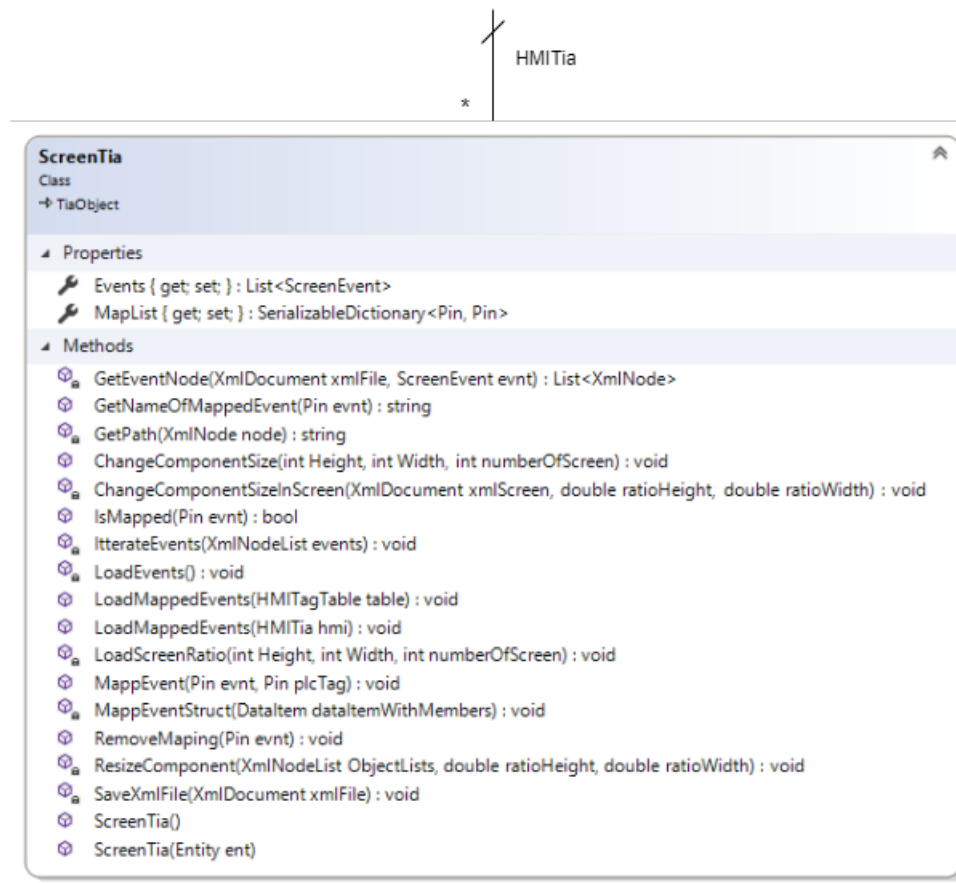
Obr. A.7: Class diagram 7. část
