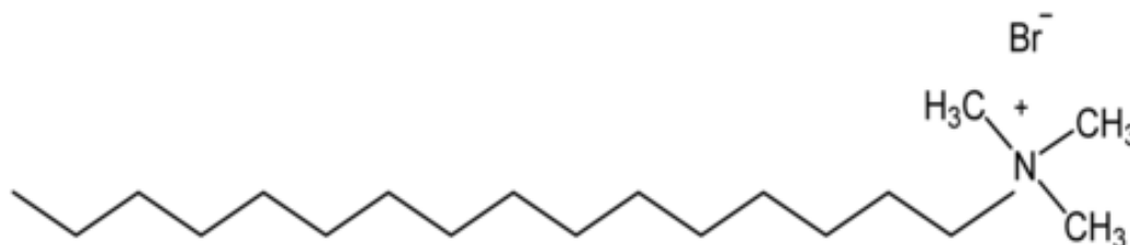
Obr.3: Štruktúra CTAB [8]
