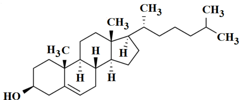
Obr.11: Štruktúra cholesterolu [22]
