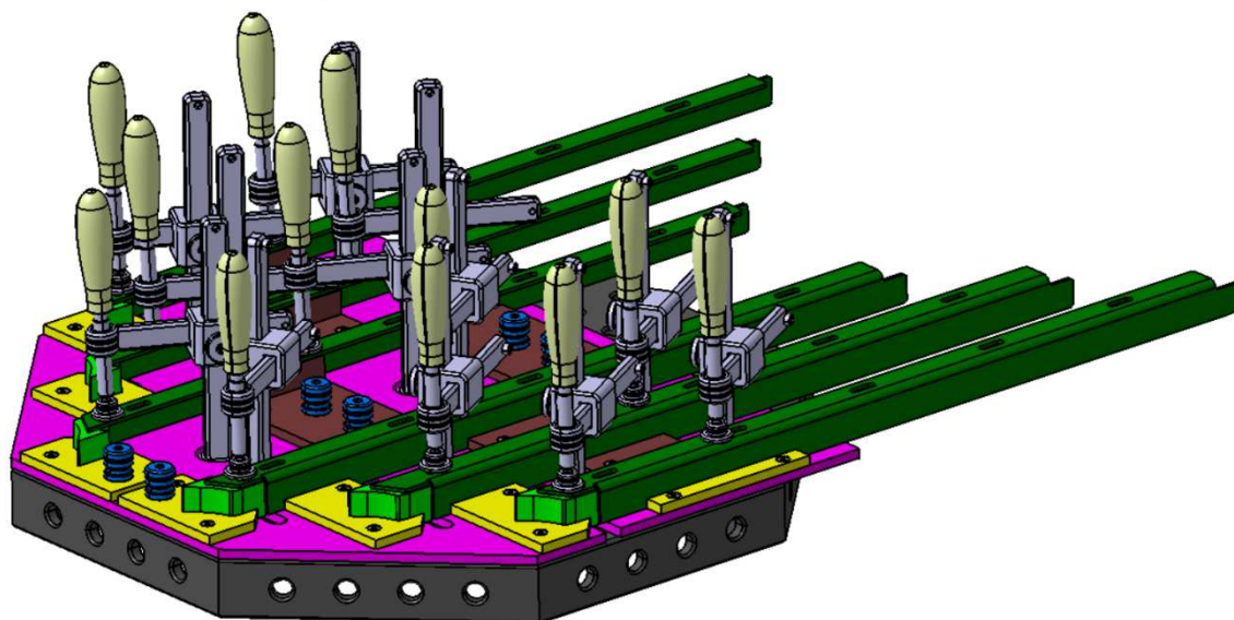
Obr. 90 Svařovací přípravek
