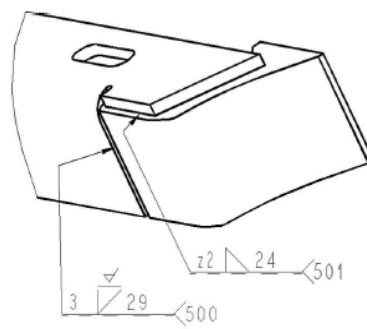
Obr. 6 svary [4]
