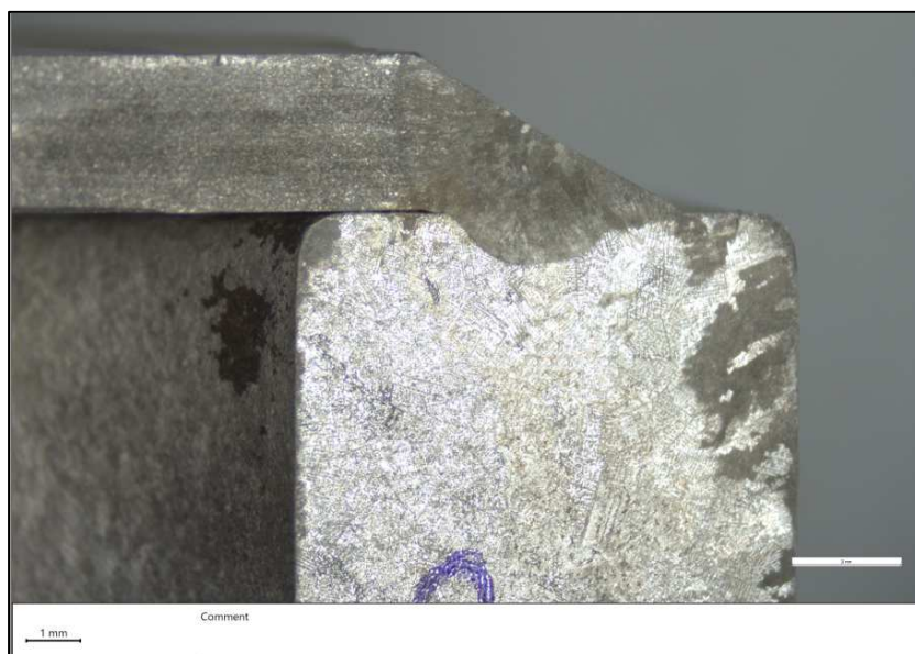
Obr. 67 Vzorek A – koutový svar z3 [4]
