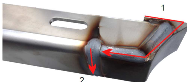
Obr. 60 Schéma tvorby svarů
