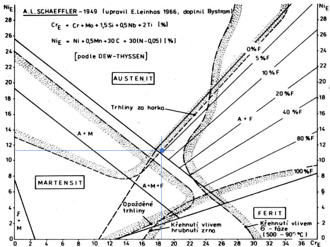
Obr. 11 Schaefflerův diagram [15]
