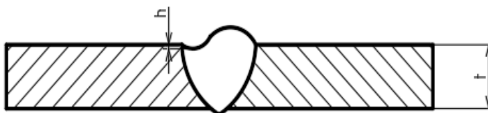
Obr. 58 Neúplné vyplnění svaru [45]
