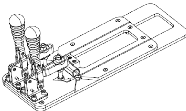
Obr. 17 Upínací přípravek [24]
