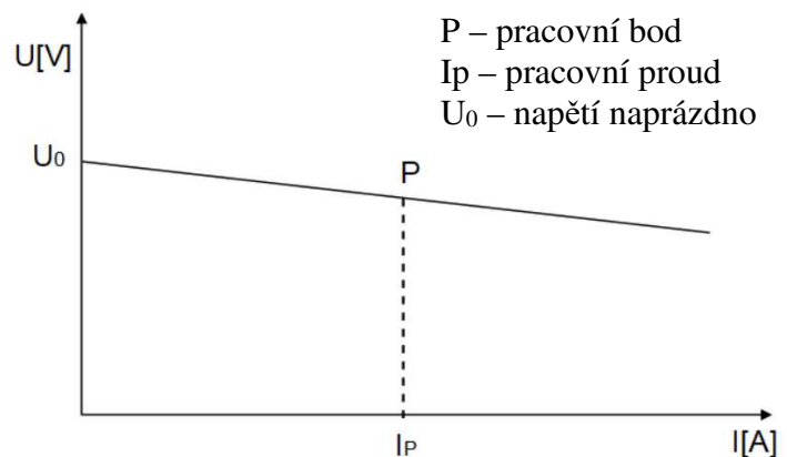
Obr. 24 plochá statická V-A charakteristika [8]
