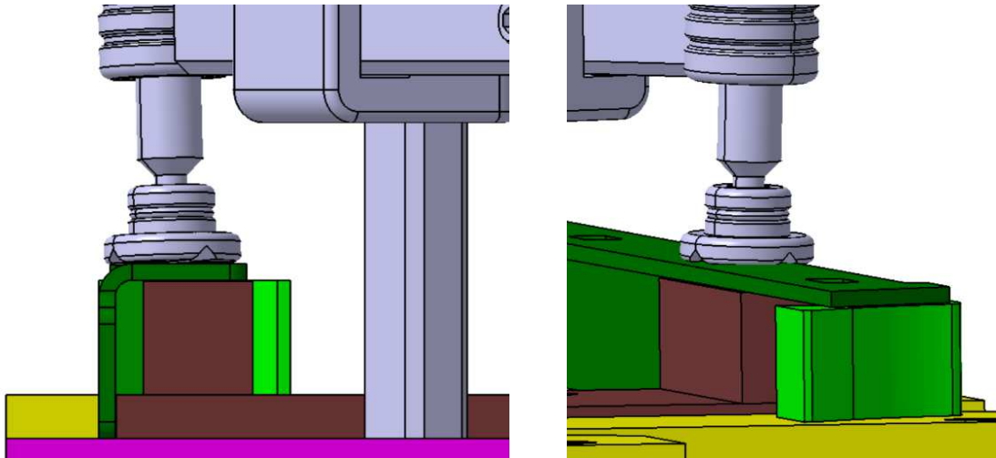
Obr. 84 Podepření kolejnice
