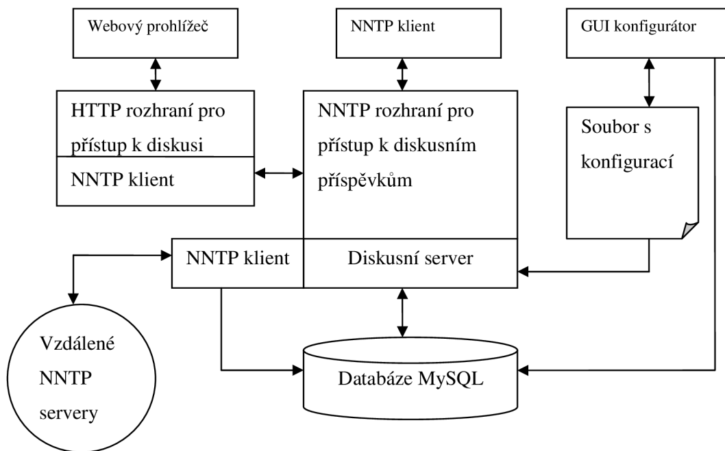
Obr. 1: Struktura aplikace
