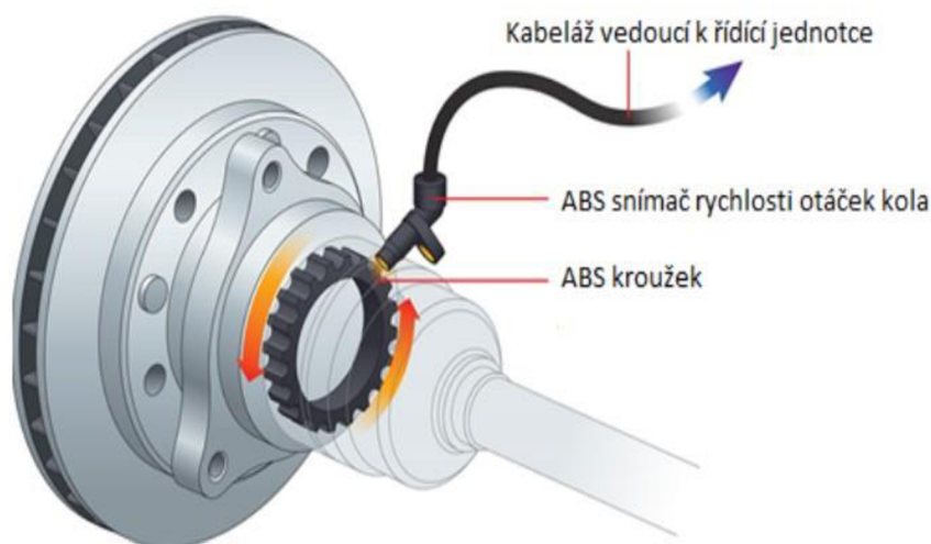
Obr. 7.: Ukázka systému ABS [14]
