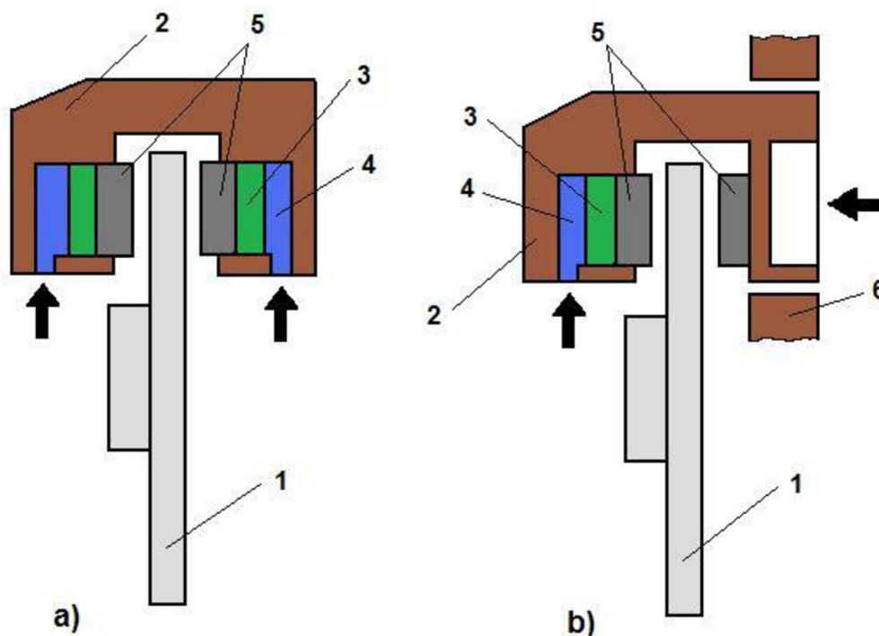
Obr. 13.: a) kotoučová brzda s pevným třmenem b) kotoučová brzda s plovoucím třmenem [21]
