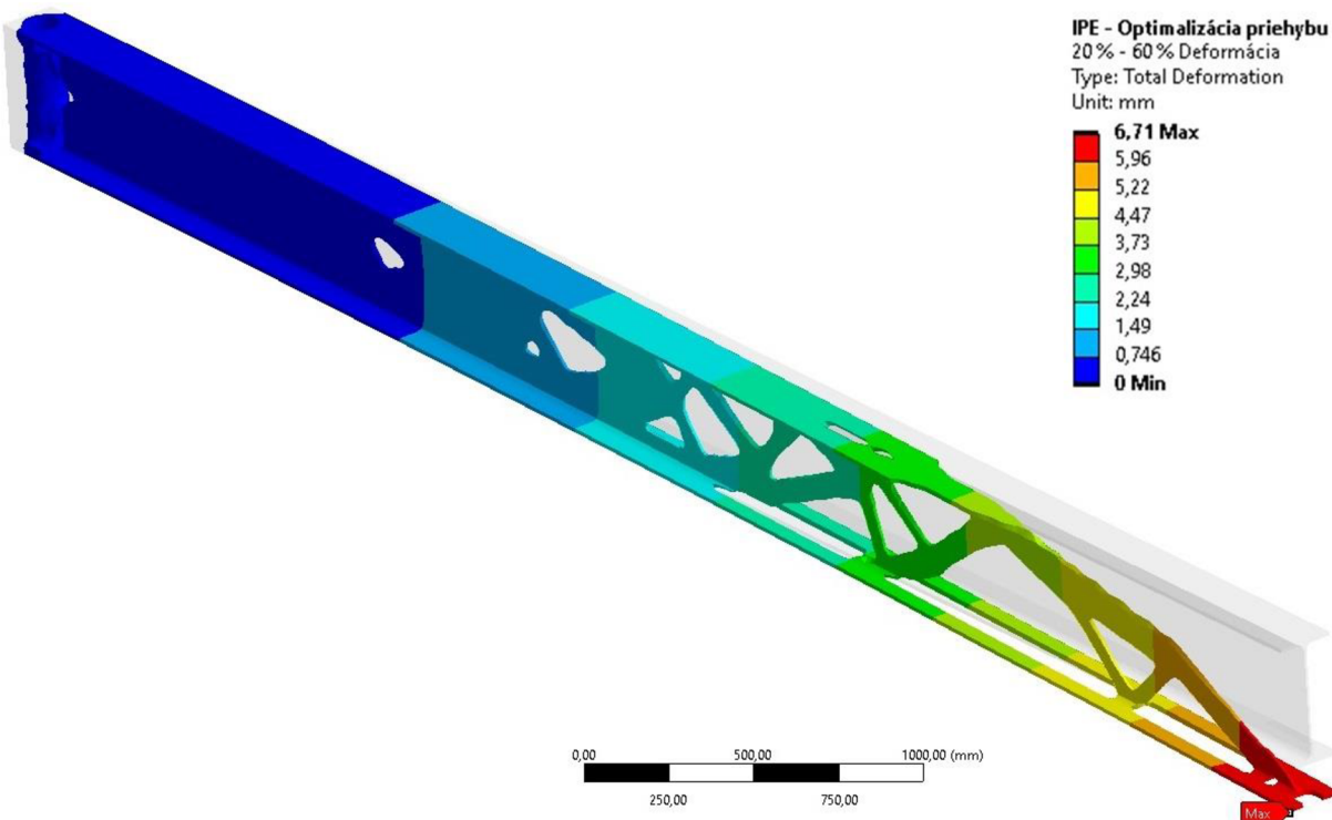
Obr. B 2 Priebeh deformácie v mm na optimalizovanom výložníku IPE profilu s cieľom optimalizácie priehtybu a mierou zachovania materiálu 20% - 60% pôvodnej hmotnosti
