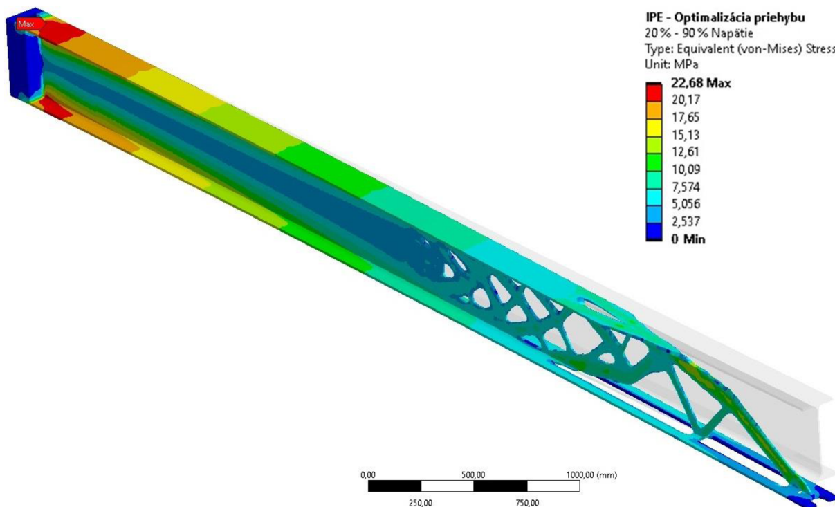
Obr. B 3 Priebek von-Mises napätia v MPa na optimalizovanom výložníku IPE profilu s cieľom optimalizácie priehybu a mierou zachovania materiálu 20% - 90% pôvodnej hmotnosti
