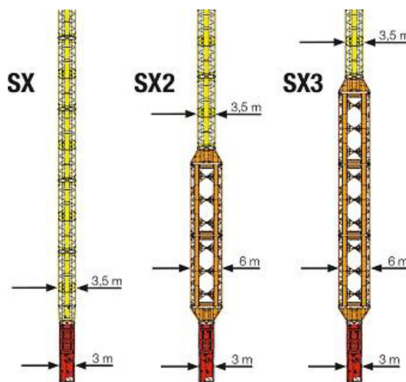
Obr. 7 Systém SX konštrukcie výložníkov firmy Liebherr [57]
