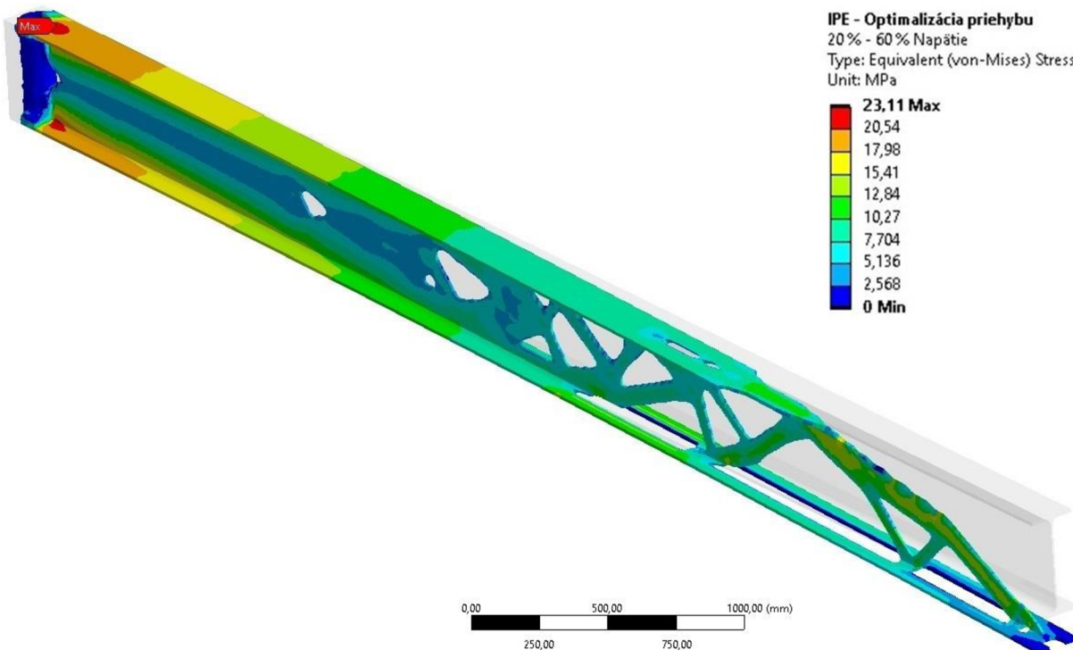
Obr. B 1 Priebeh von-Mises napätia v MPa na optimalizovanom výložníku IPE profilu s cieľom optimalizácie priehtybu a mierou zachovania materiálu 20% - 60% pôvodnej hmotnosti
