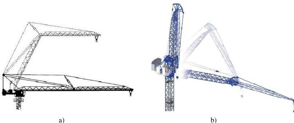
Obr. 6 Lomený výložník s 2. výložníkovou časťou: a) vodorovnou, b) sklopnou [58],[51]
