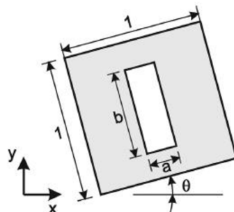
Obr. 27 Základná štvorcová bunka s obdĺžnikovou mikrodutinou [4]
