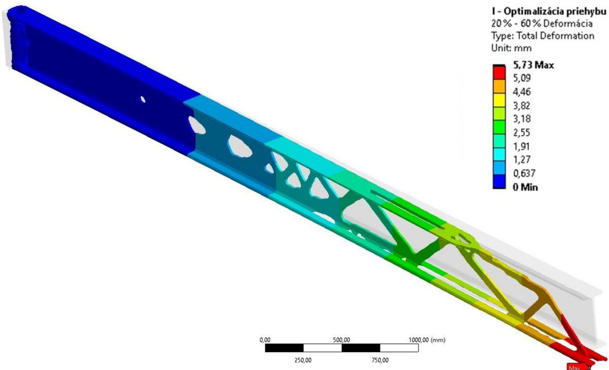
Obr. B 6 Priebeh deformácie v mm na optimalizovanom výložníku I profilu s cieľom optimalizácie priehybu a mierou zachovania materiálu 20 % - 60 % pôvodnej hmotnosti
