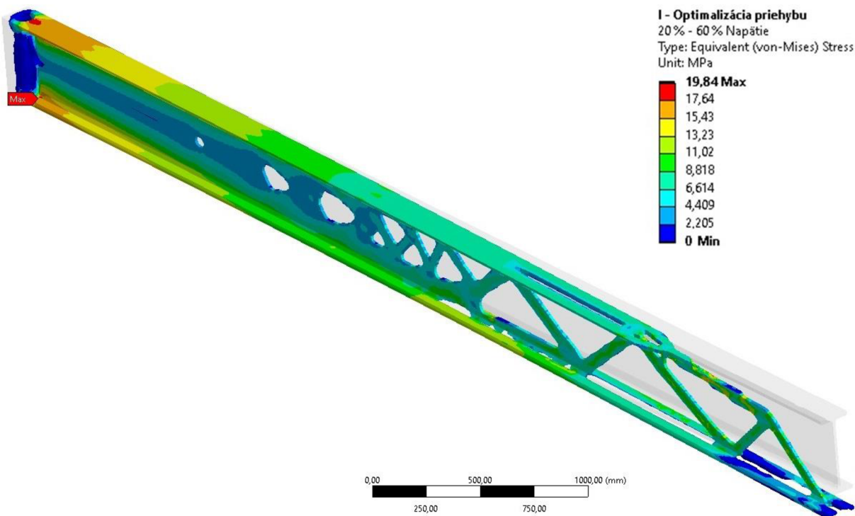
Obr. B 5 Priebeh von-Mises napätia v MPa na optimalizovanom výložníku I profilu s cieľom optimalizácie priehybu a mierou zachovania materiálu 20 % - 60 % pôvodnej hmotnosti
