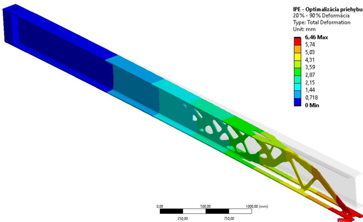
Obr. B 4 Priebek deformácie v mm na optimalizovanom výložníku IPE profilu s cieľom optimalizácie priehybu a mierou zachovania materiálu 20% - 90% pôvodnej hmotnosti
