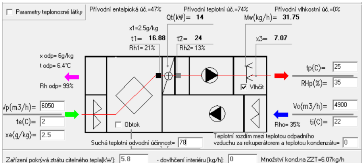
Obr. 27 Parametry jednotky při rozdílu teplot 20 K – z.č. 3 Remak
