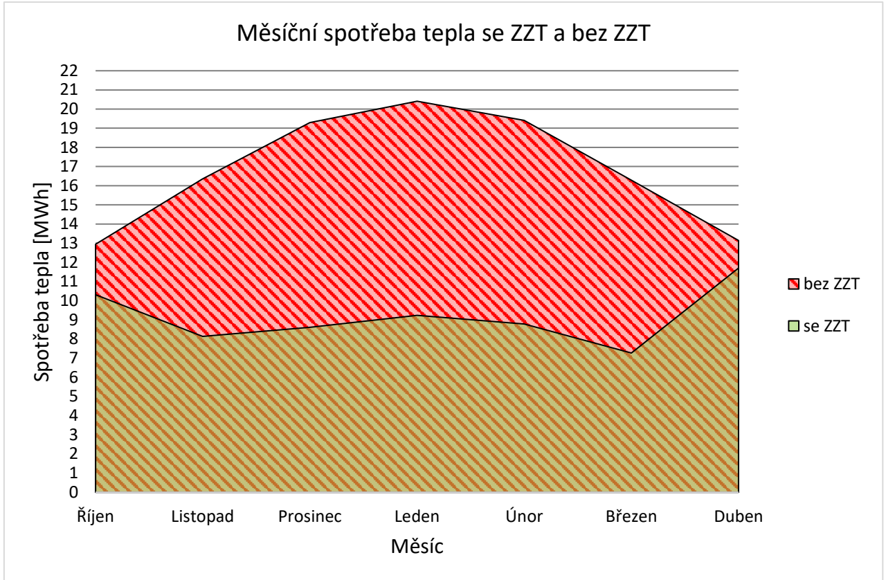
Graf 9 Měsíční spotřeby tepla se ZZT a bez ZZT – z.č. 4 Janka
