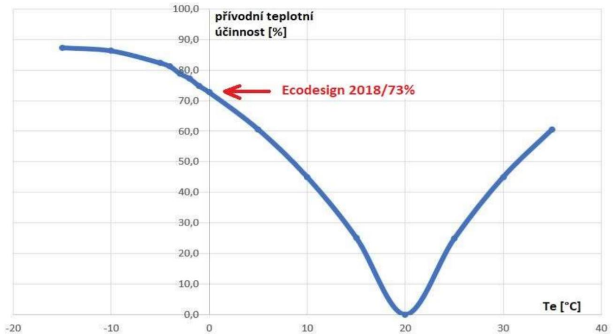
Graf 4 Závislost účinnosti ZT na venkovní teplotě [20]
