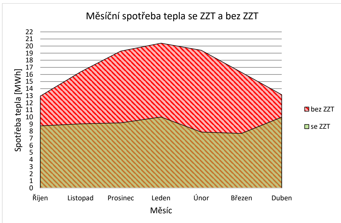
Graf 12 Měsíční spotřeby tepla se ZST a bez ZST – z.č. 4 Remak
