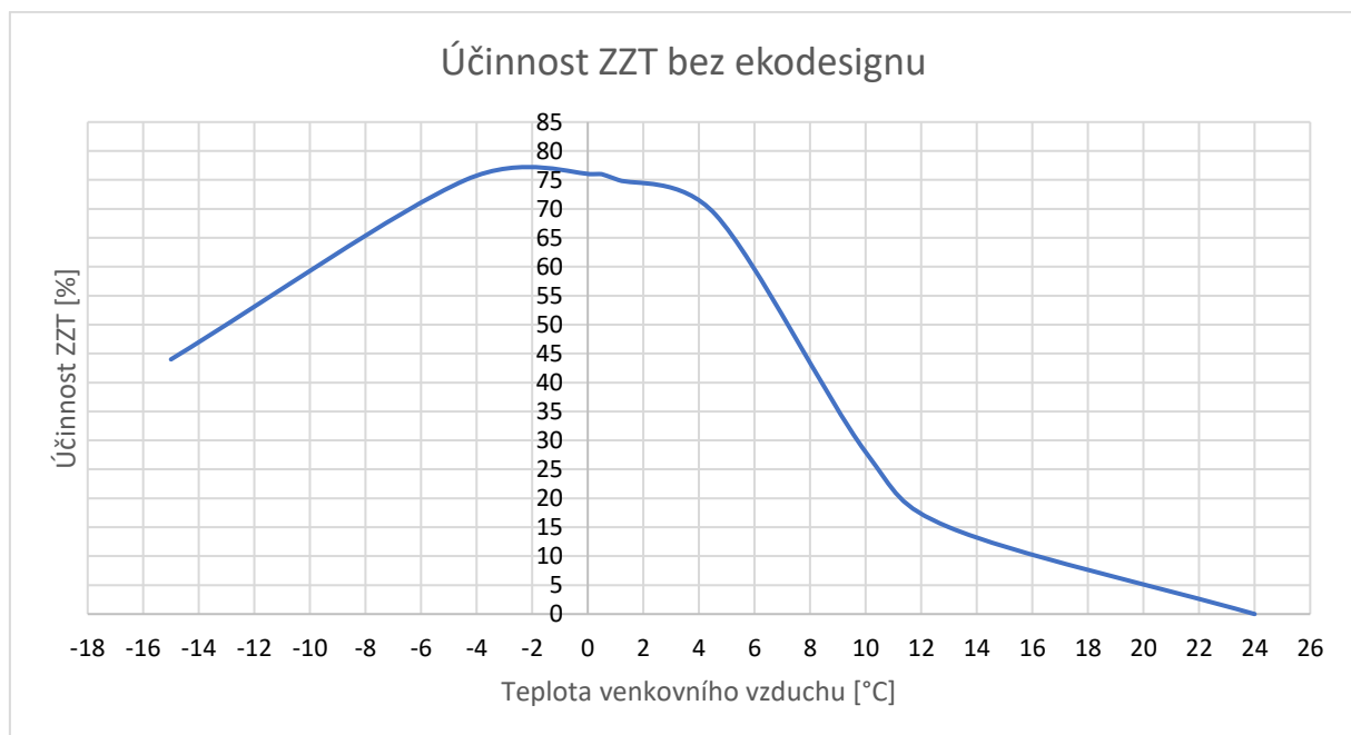
Graf 1 Závislost účinnosti ZZT na venkovní teplotě vzduchu (bez ekodesignu)
