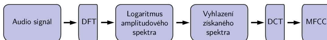
Obr. 5.7: Blokové schéma výpočtu Melovských keprálních koeficientů
