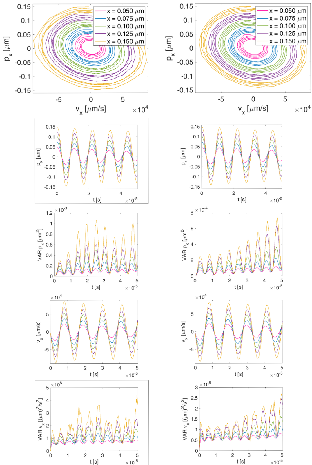
Příloha 06: Fázové portréty a další momenty – osa x, 20 Pa.
