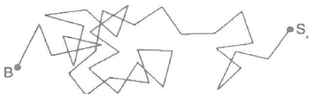
Obr. 2.1 Trajektorie Brownova pohybu
