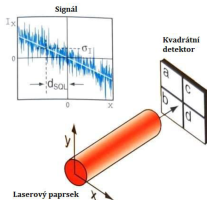
Obr. 3.2 Mechanismus zisku polohových souřadnic částice
