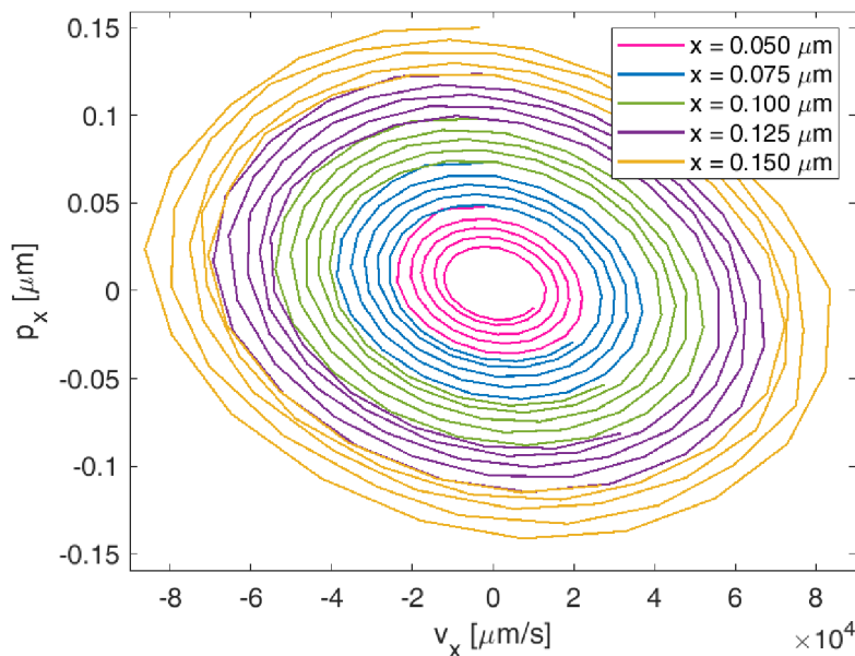
Obr. 4.7 Fázový portrét
