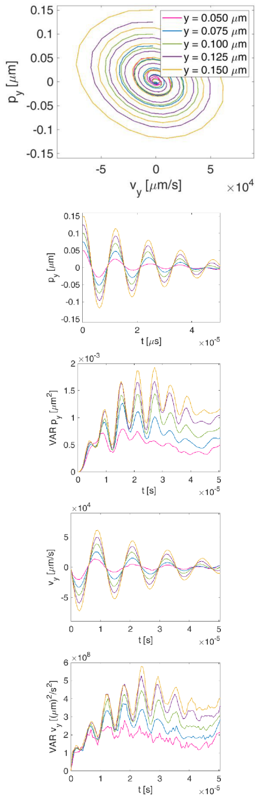
Příloha 26: Fázové portréty a další momenty – osa y, 1000 Pa.
