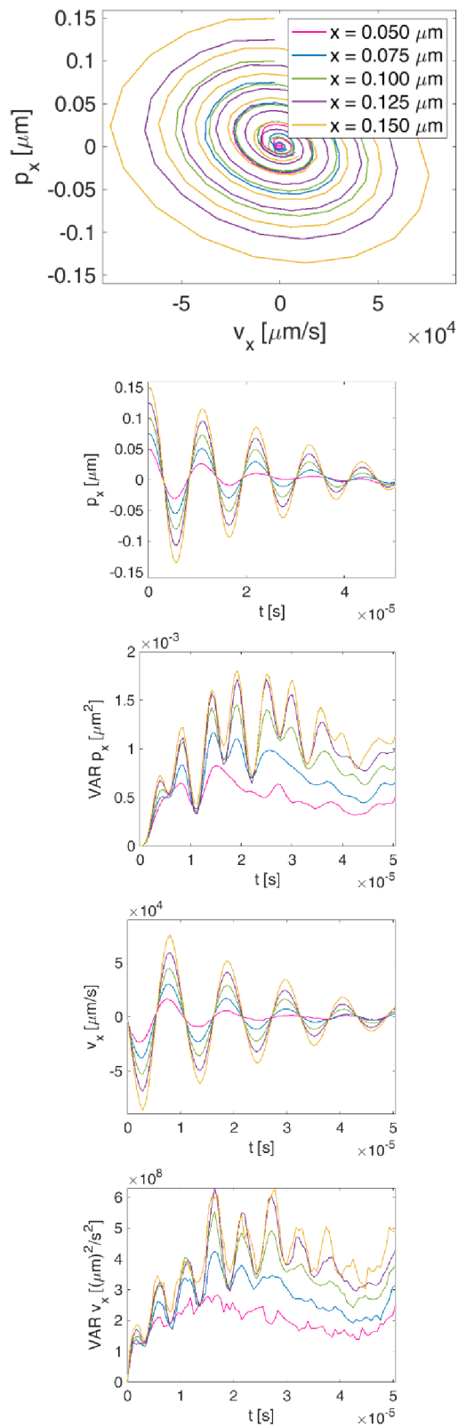
Příloha 14: Fázové portréty a další momenty – osa x, 1000 Pa.
