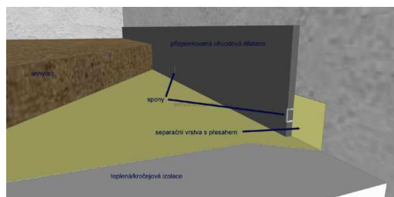
obr. 7.1.6b. Přispokování Mirelonu
