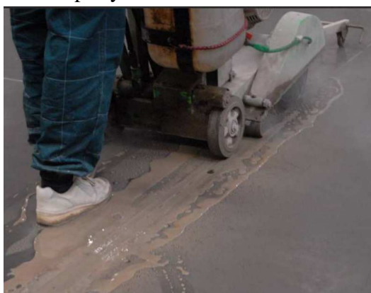
Obr. 7.6b. Prořezávání spár
