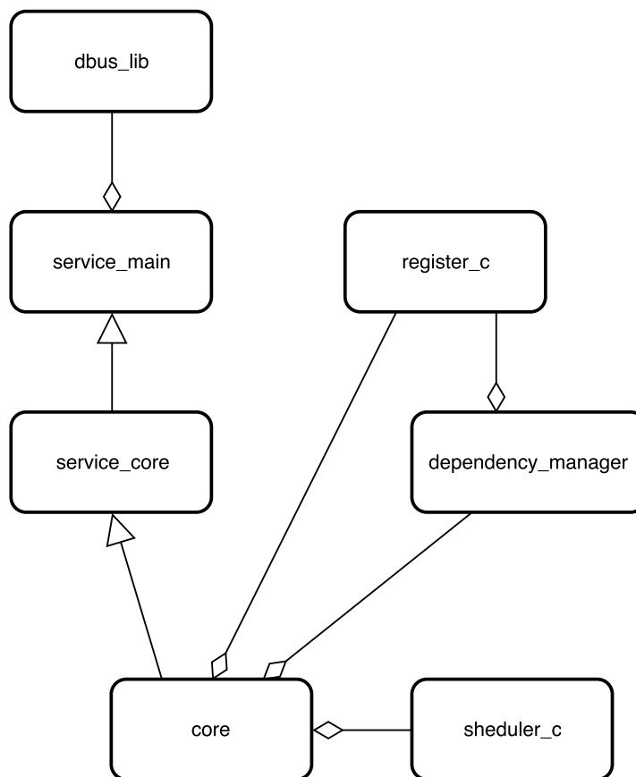
Obrázek 3.2: Hierarchie tříd
