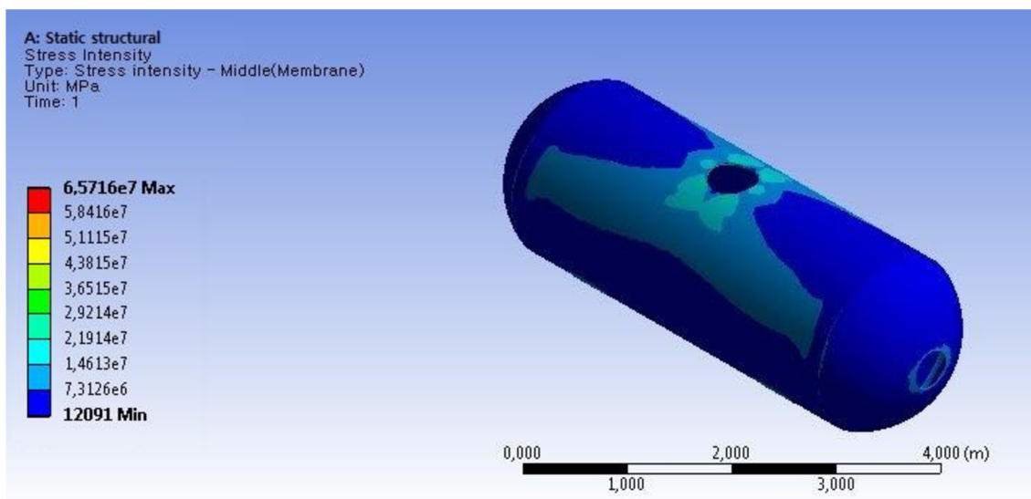
Obr. 6.3 Membránové napětí
