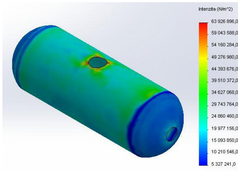
Obr. 5.6 Membránové napětí
