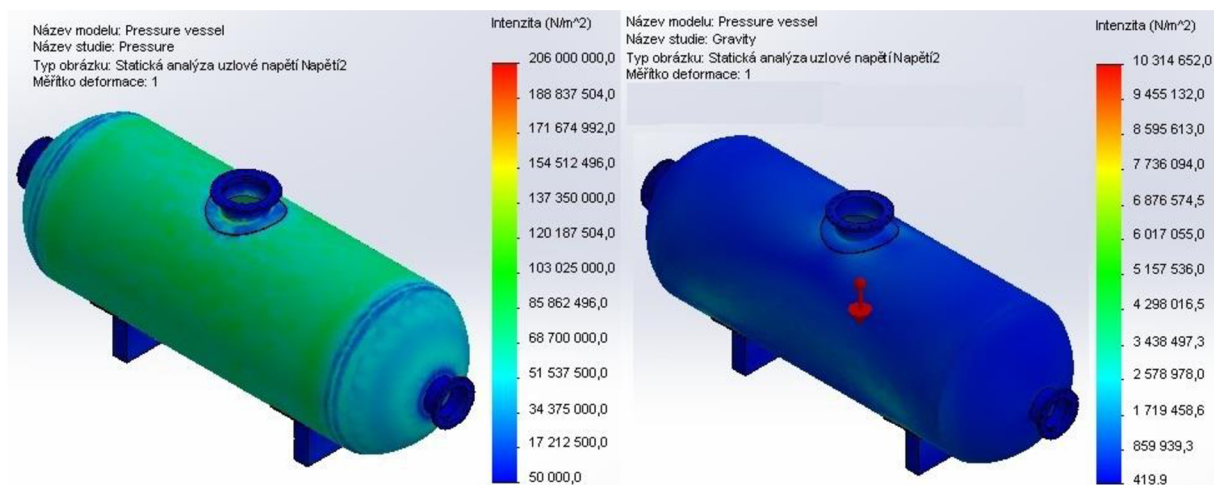
Obr. 5.5 Grafické zobrazení výsledných napětí jednotlivých analýz (zleva: tlakové namáhání, gravitace)
