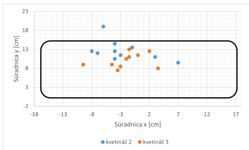
Graf 8 – Polohy koncového efektora nad obdĺžnikovými kvetináčmi
