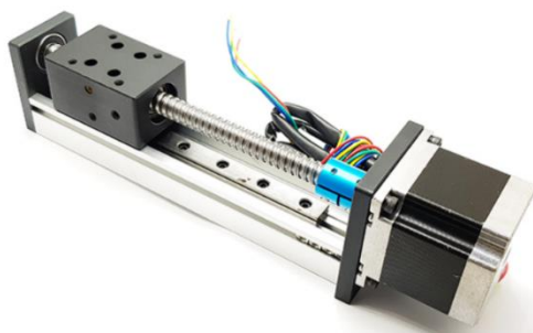
Obrázok 12.10 – Lineárny pojazd s guľočkovou skrutkou a krokovým motorom, [31]
