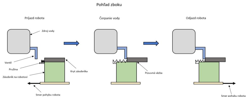
Obrázok 5.5 – Schéma zabezpečenia transferu vody do zásobníka otvorením a zatváraním krytu s pružinou
