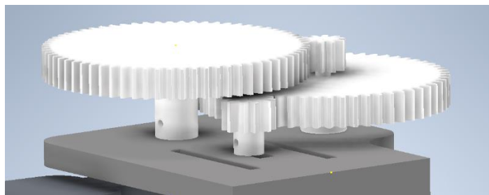
Obrázok 7.3 – Detail modelu ozubeného súkolia vytvoreného v programe Inventor
