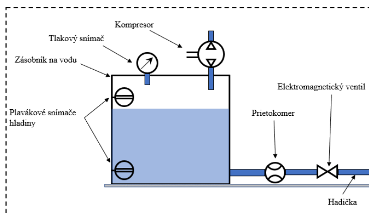
Obrázok 4.13 – Schéma variantu vodného okruhu s jedným kompresorom
