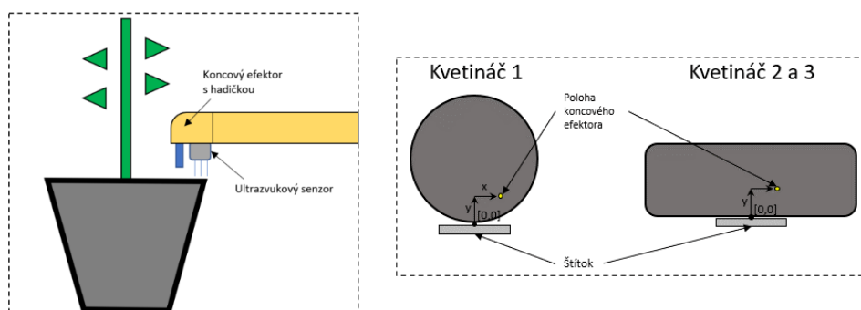
Obrázok 8.6 – Vľavo: detail koncového efektora ramena nad priestorom kvetináča, vpravo: typy testovaných kvetináčov a spôsob merania polohy koncového efektora
