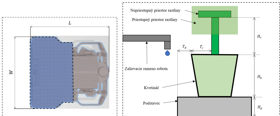
Obrázok 3.1 – Schematické zakreslenie rozmerov robota Breach [6] a rozmerových parametrov modulu a kvetináča [1]
