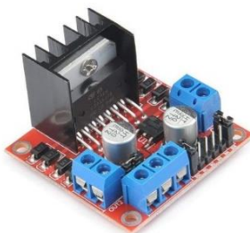
Obrázok 12.21 – H most L298N, [45]
