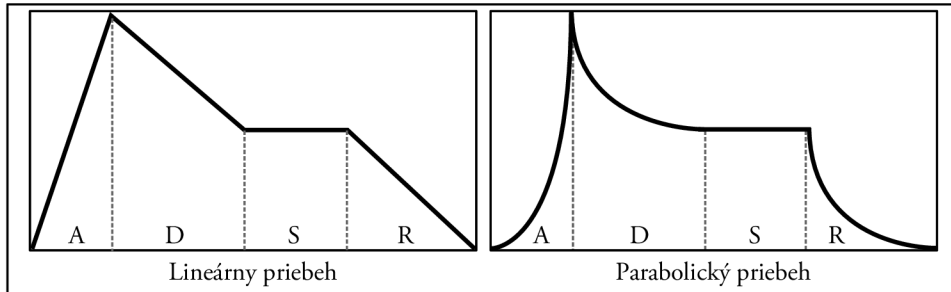
Obr. 6.3: Tvary modulačnej obálky pre zosilňovač a filter
