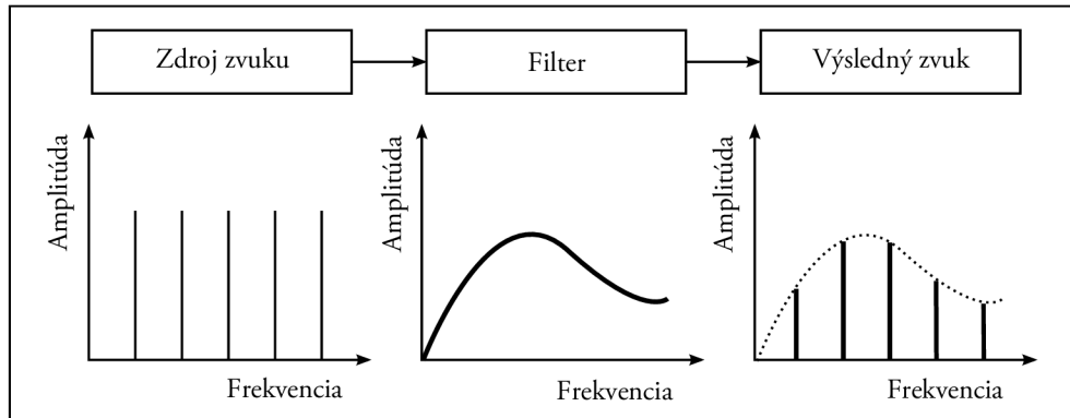
Obr. 2.2: Bloková schéma rozdielovej syntézy
