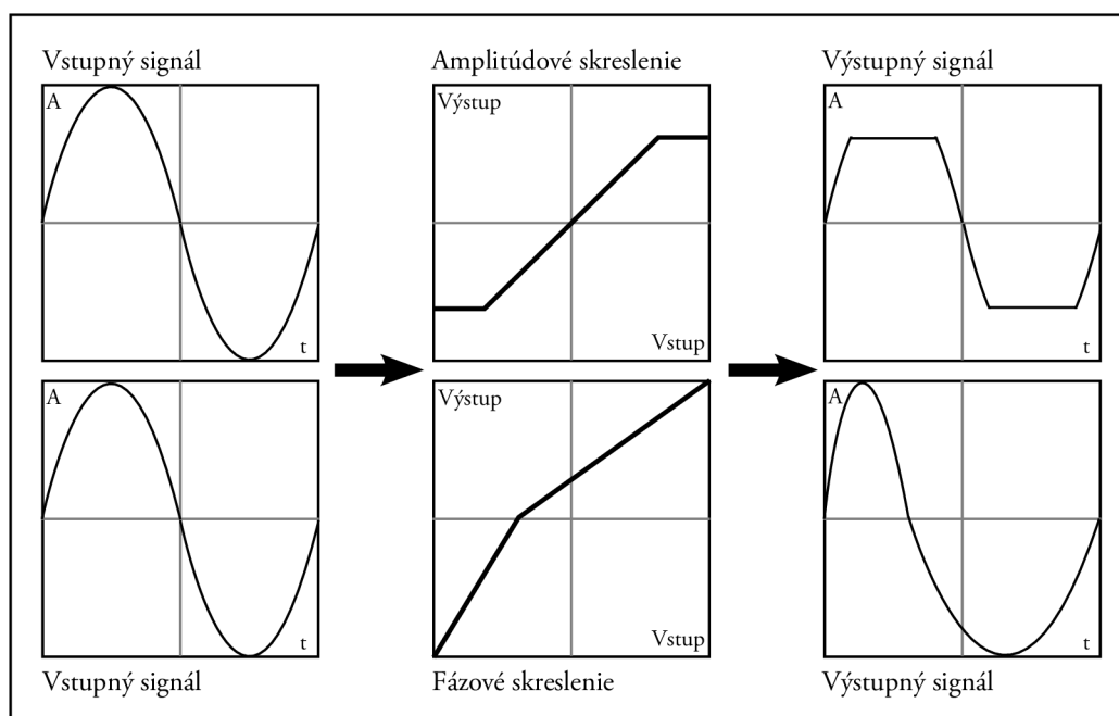
Obr. 2.4: Znázornenie amplitúdovej a fázovej tvarovej syntézy
