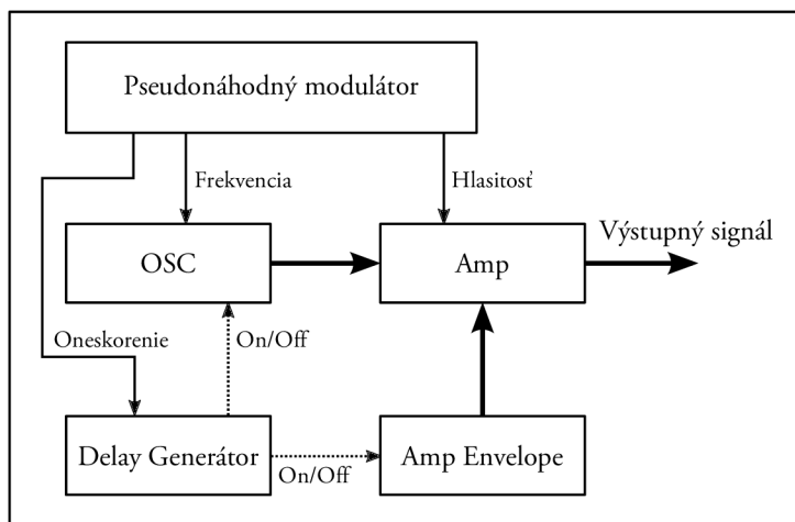
Obr. 7.1: Bloková schéma granulárneho modulu
