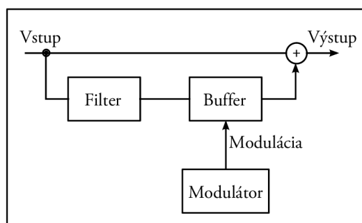
Obr. 7.7: Bloková schéma efektu Chorus
