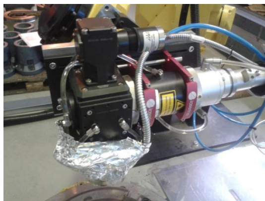
Obr. 36 Laserová kalící hlava
