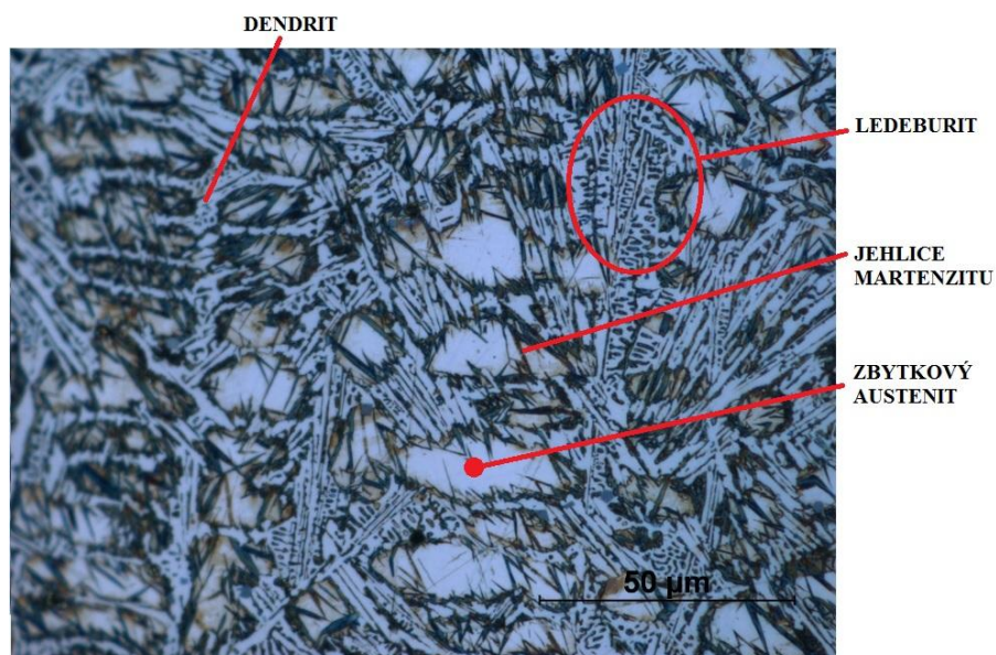
Obr. 58 Detail struktury bílé litiny, zvětšeno 1000x
