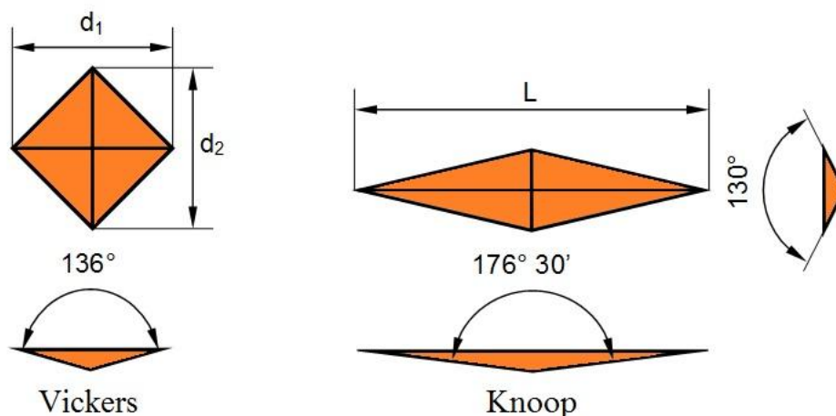
Obr. 32 Vtisk dle Vickerse a Knoopa [58]
