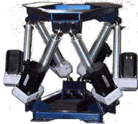
Obr. 4.11: Simulační plošina firmy Pragolet [24].
