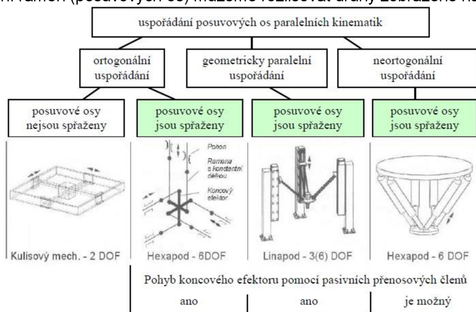
Obr. 2.5: Rozdělení paralelních mechanismů z hlediska uspořádání ramen [1].
