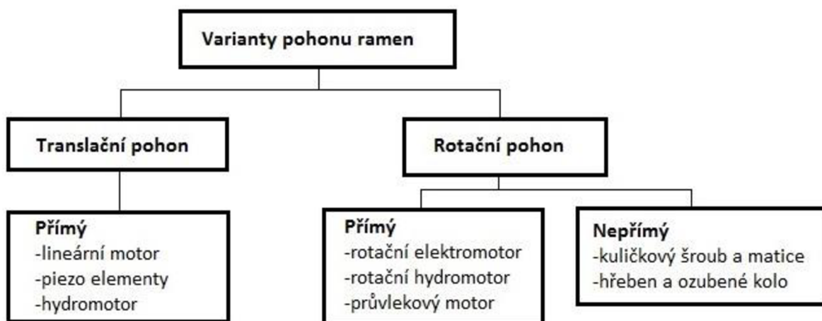
Obr. 2.6: Rozdělení pohonů servoramen [1].
