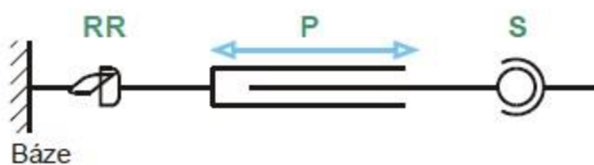
Obr. 2.4: Uspořádání kloubů ve vodícím řetězci [1].
