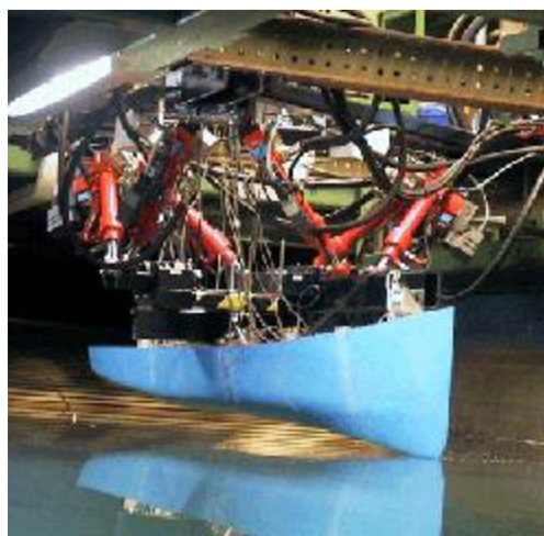
Obr. 4.12: Hexapod Hexamove testující trup lodí [25].
