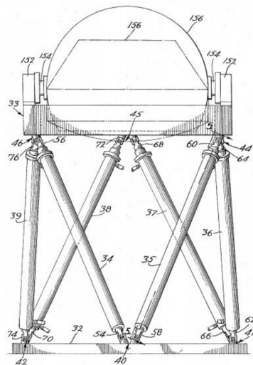
Obr. 1.6: Návrh Cappelova leteckého simulátoru [8].
