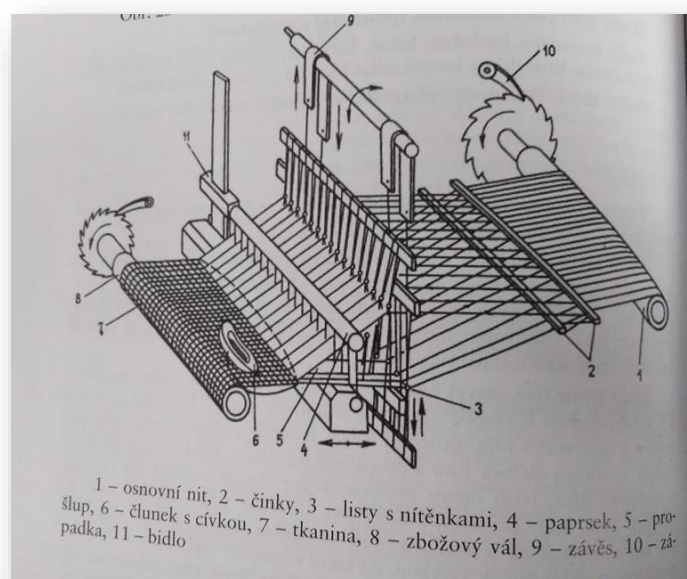
Obr. č. 3 – Ukázka tkalcovského stavu s popisem jednotlivých částí
