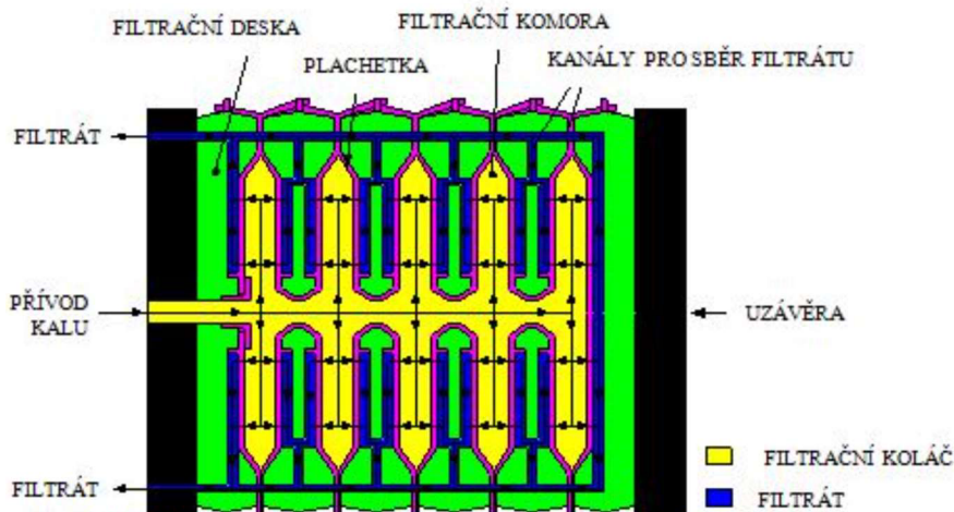
Obr. 18. Průřez filtrem kalolisu (CIF, 2024)
