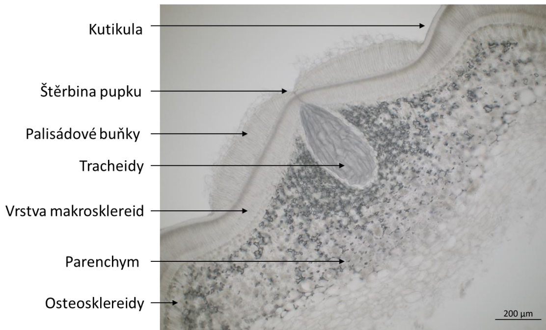
Obr. 3: Struktura osemení v oblasti pupku planého, dormantního genotypu JI64 ve stádiu 16 DAP (DAP – day after polination).
