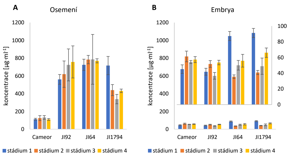
Obr. 12: Koncentrace celkových fenolů v osemení (A) a embryích (B) semen hrachu genotypu Cameor, JI92, JI64 a JI1794 ve čtyřech vývojových stádiích.
