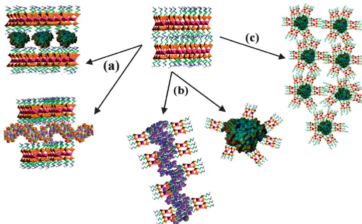
Obrázek 3.1: Příprava bionanokompozitů: (a) vmezeření proteinů či DNA do struktury aminojílu, (b) obalování jednotlivých záporně nabitých biopolymerů či klastrů, (c) syntéza částečně uspořádaných nadstruktur [3]
