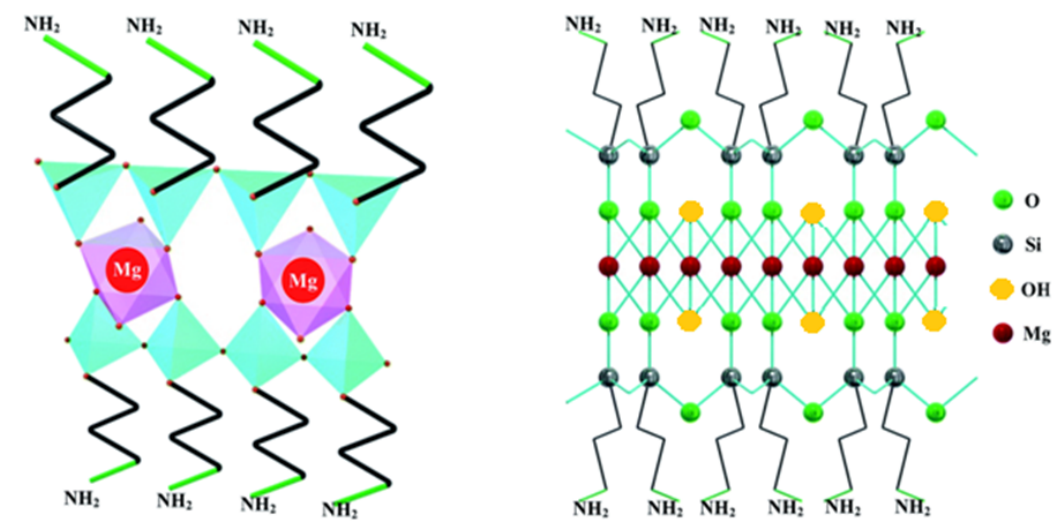
Obrázek 2.3: Struktura aminojílu [11]
