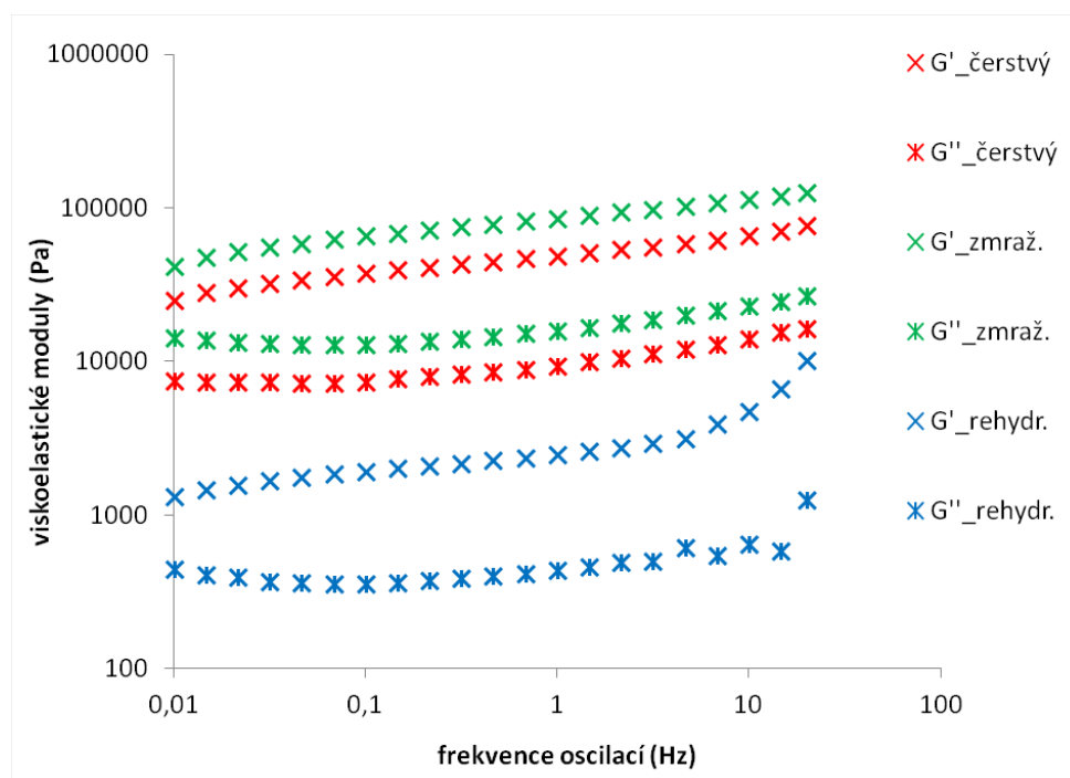
Obrázek 6.16: Závislost viskózního G'' a elastického modulu G' na frekvenci oscilací pro vzorek čerstvého, rehydratovaného a rozmraženého hydrogelu Aj-HyA (MMW)
