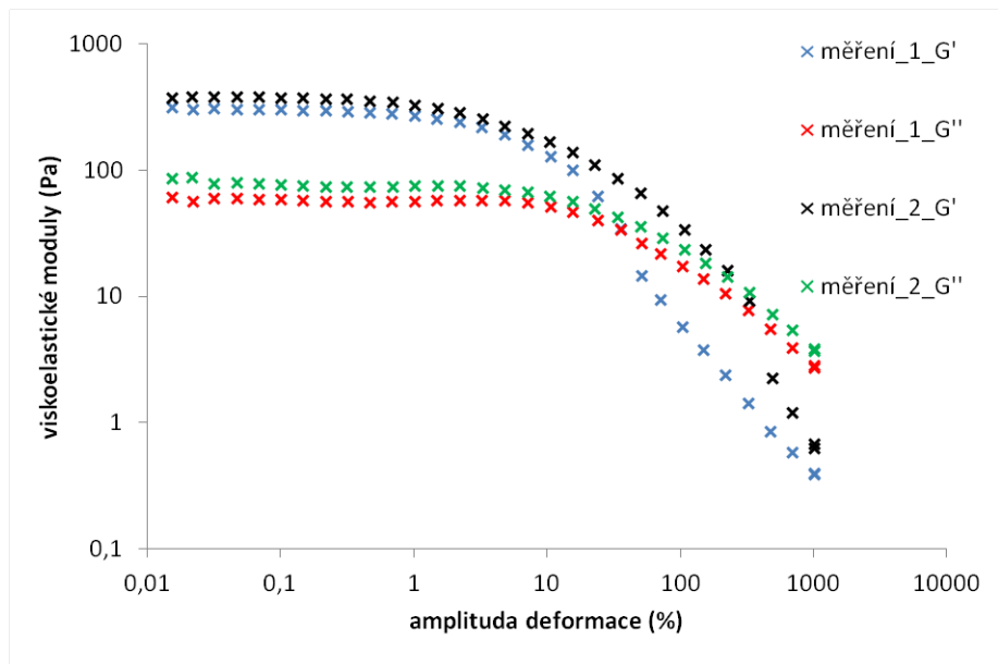
Obrázek 10.5: Měření závislosti ztrátového a paměťového modulu na amplitudě deformace pro čerstvý vzorek hydrogelu Aj-HyA (MMW)
