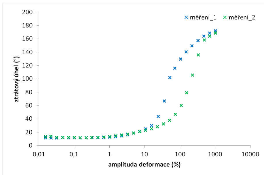
Obrázek 10.6: Závislost ztrátového úhlu na amplitudě deformace pro čerstvý vzorek hydrogelu Aj-HyA (MMW)
