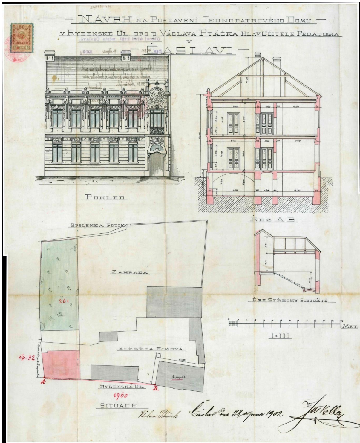
(R – III – F/3 Plány Husova asylu)
